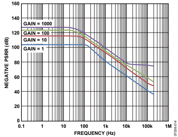
图24.负PSRR与频率的关系
