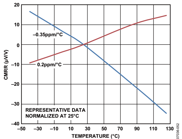
图32. 共模抑制比(CMRR)与温度的关系, G=1
