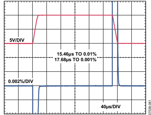
图48. 大信号脉冲响应与建立时间的关系 ( G = 10 , 10 V步进, V_S = \pm 15 V)
