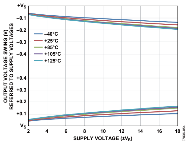
图34.输出电压摆幅与电源电压的关系 (RL = 10 kΩ)
