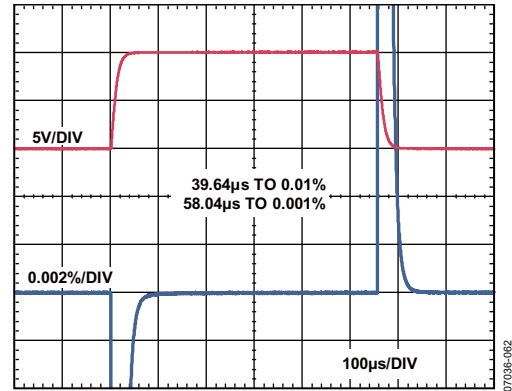
图49. 大信号脉冲响应与建立时间的关系 ( G = 100 , 10 V步进, V_S = \pm 15 V)
