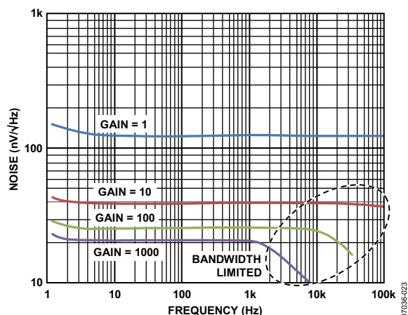
图42.电压噪声谱密度与频率的关系
