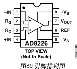
图60.引脚排列图
