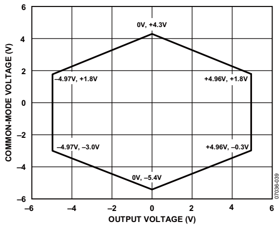
图11.输入共模电压与输出电压的关系， 双电源供电， V_S = +5V , G = 1
