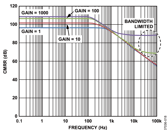
图28. CMRR与频率的关系 (RTI, 1 kΩ非均衡电源)
