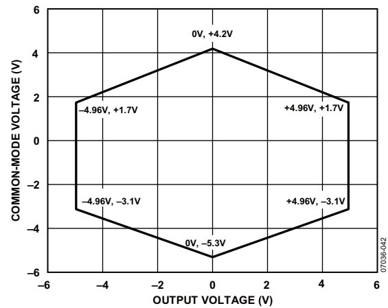
图14.输入共模电压与输出电压的关系， 双电源供电， V_S = +5V , G = 100
