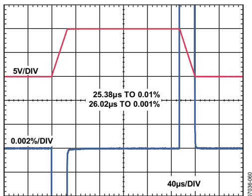
图47. 大信号脉冲响应与建立时间的关系 ( G = 1 , 10 V步进, V_S = \pm 15 V)
