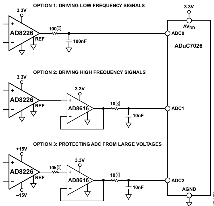
图66.驱动ADC
