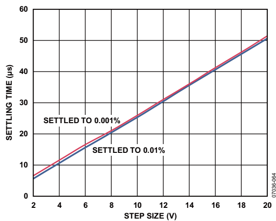
图56.建立时间与步长的关系 ( V_S = \pm 15 V 双电源供电)
