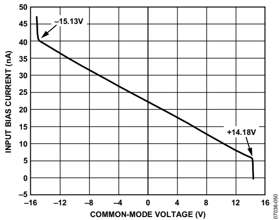
图22.输入偏置电流与共模电压的关系, V_S = +15V
