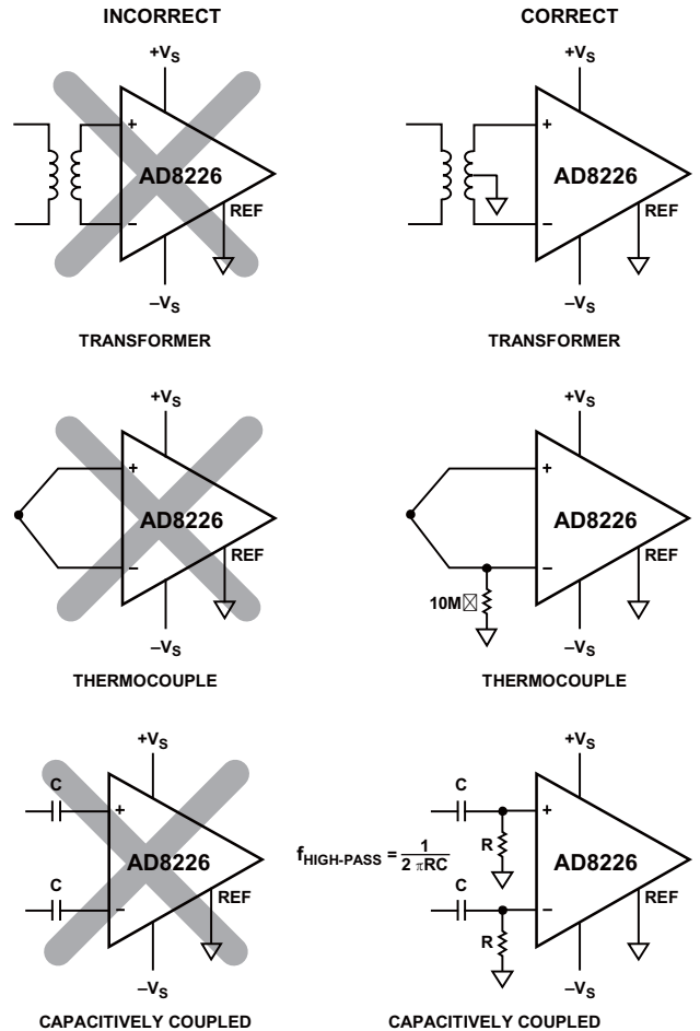
图62. 创建一条 I_{BIAS} 返回路径
