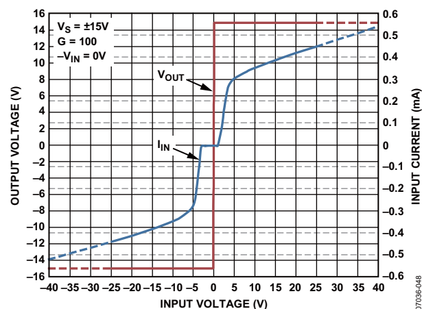
图20.输入过压性能， G = 100 ， V_S = 15\text{ V}
