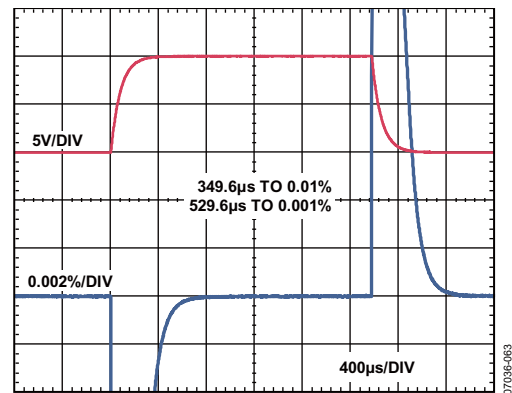
图50. 大信号脉冲响应与建立时间的关系 ( G = 1000 , 10 V步进, V_S = \pm 15 V)
