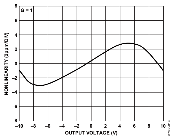
图38.增益非线性度 (G = 1, RL ≥ 2 kΩ)
