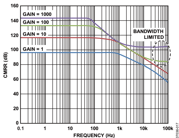
图27. CMRR与频率的关系 (RTI)
