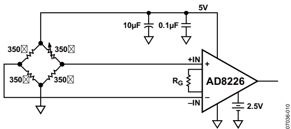
图65.精密应变计
