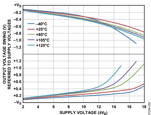
图35.输出电压摆幅与电源电压的关系 (RL = 2 kΩ)
