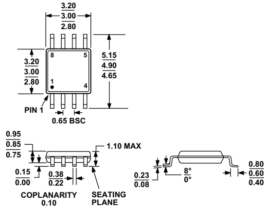
图67. 8引脚超小型封装[MSOP] (RM-8)
