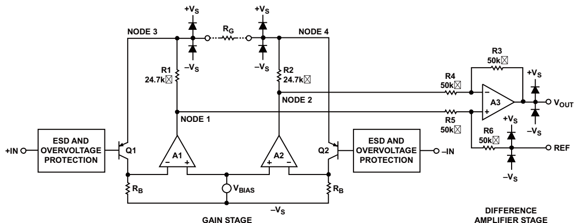
图58.简化原理图
