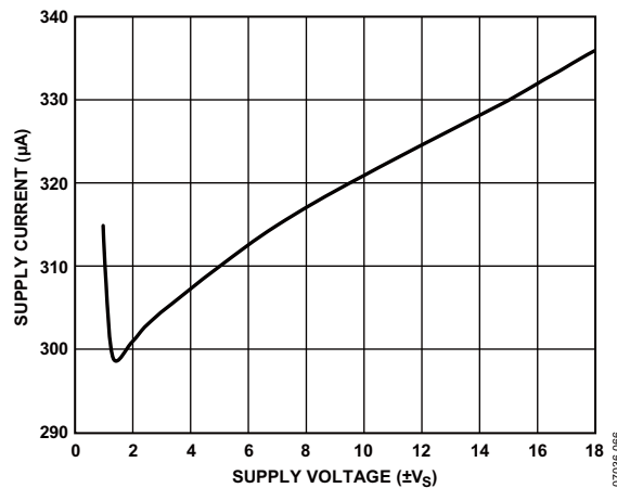
图57.电源电流与电源电压的关系
