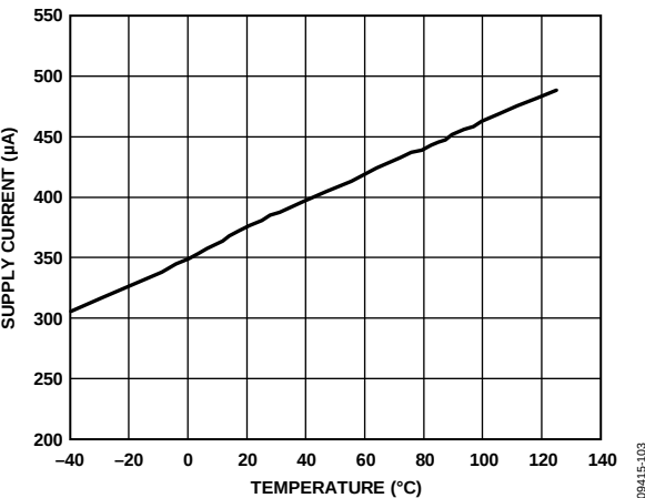
图10. 典型电源电流在温度范围内的变化( V_s = 5\text{ V} )
