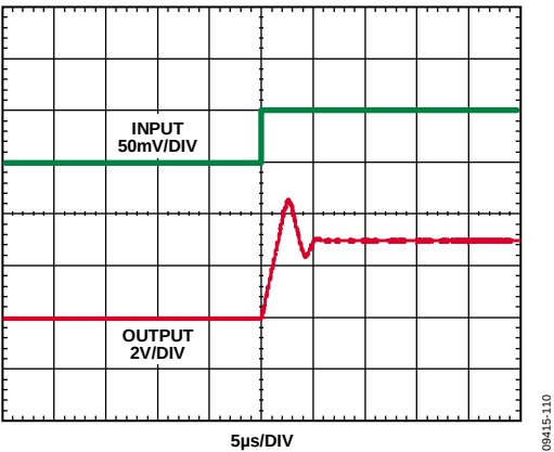
图12. 上升时间(差分输入 = 50 mV)
