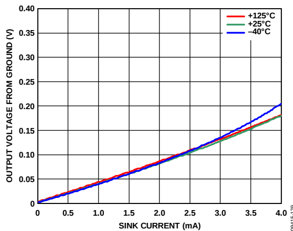
图20. 地输出电压范围与输出吸电流的关系( V_s = 5\text{ V} )
