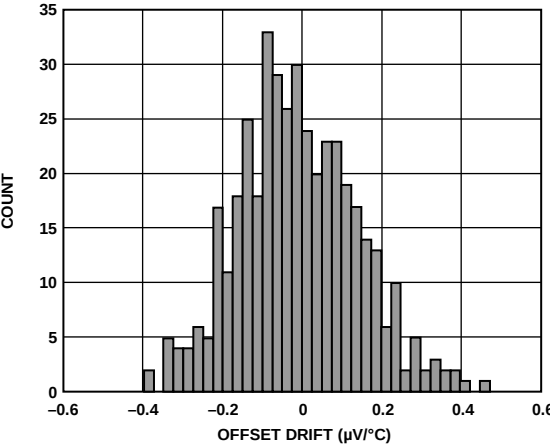
图25. 输入失调漂移分布图
