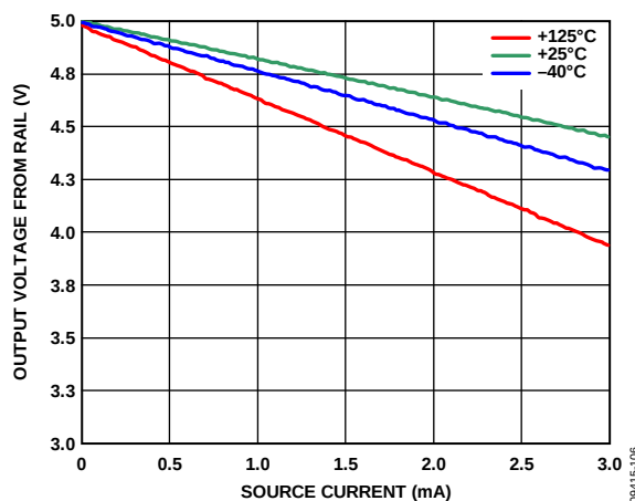
图19. 输出电压范围与输出源电流的关系( V_s = 5\text{ V} )
