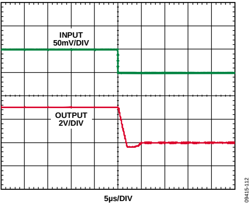
图14. 下降时间(差分输入 = 50 mV)
