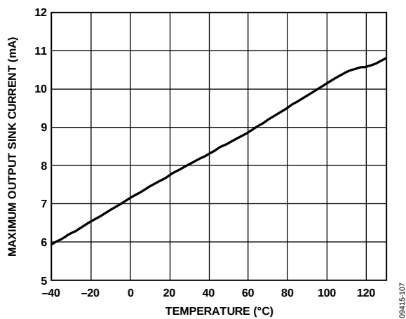
图17. 最大输出吸电流与温度的关系
