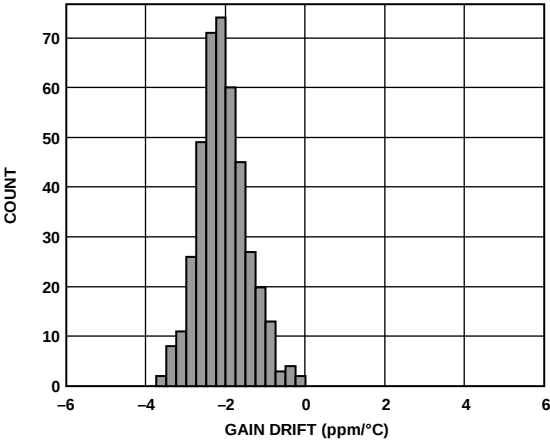
图24. 增益漂移分布图
