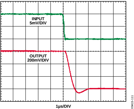
图13. 下降时间(差分输入 = 5 mV)
