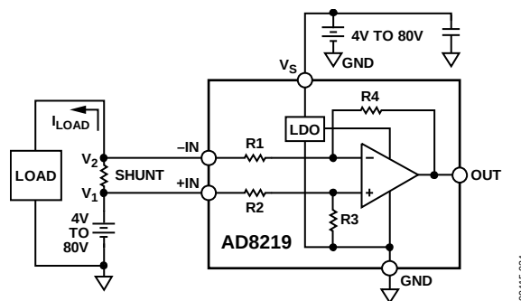
图26. 简化原理图
