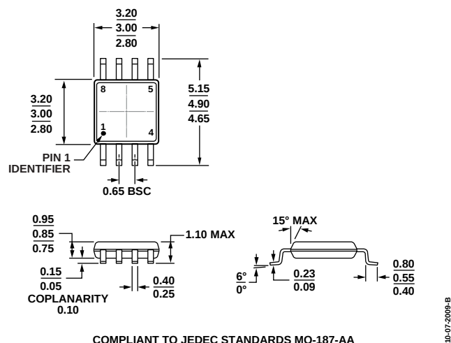
图31. 8引脚超小型封装[MSOP] (RM-8) 图示尺寸单位: mm
