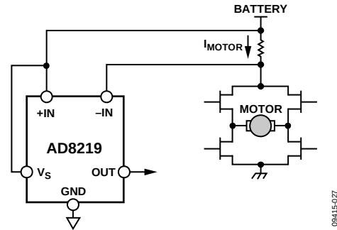
图30. 电机控制中的高端电流检测
