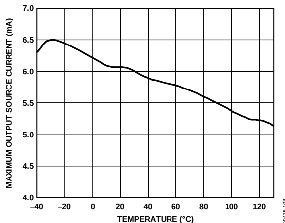
图18. 最大输出源电流与温度的关系
