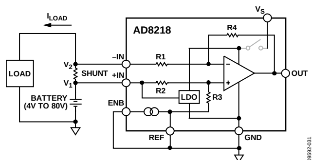
图31. ENB引脚接地的单向操作
