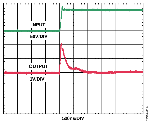
图21. 共模阶跃响应(上升)
