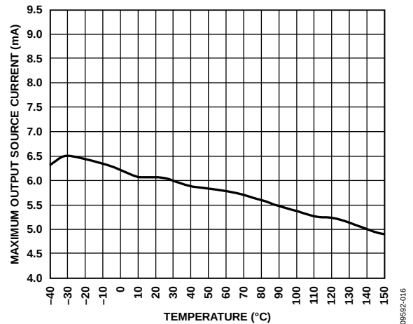
图18. 最大输出源电流与温度的关系
