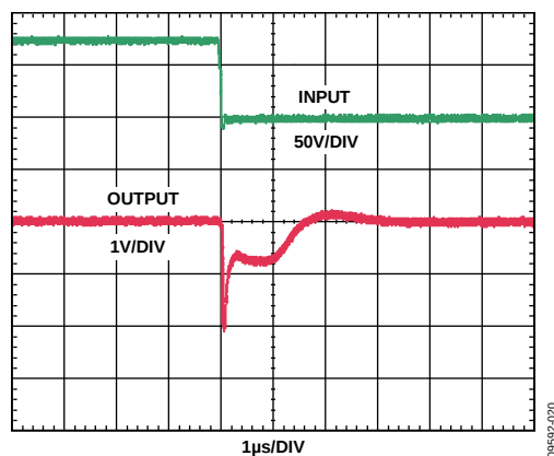
图22. 共模阶跃响应(下降)
