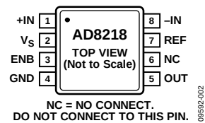
图2. 引脚配置
