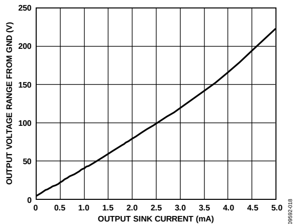
图20. GND输出电压范围与输出吸电流的关系
