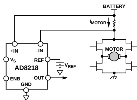
图35. 电机控制中的高端电流检测
