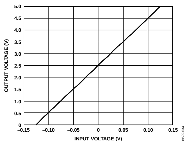
图34. 采用2.5V基准电压输入时的传递函数
