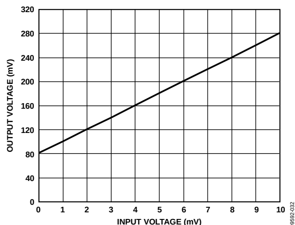
图32. ENB接地时的输出传递函数
