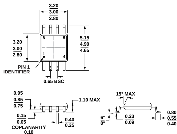
图36. 8引脚超小型封装[MSOP] (RM-8)
