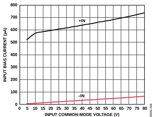
图8. 输入偏置电流与输入共模电压的关系 (差分输入电压 = 5 mV, V_s = NC )
