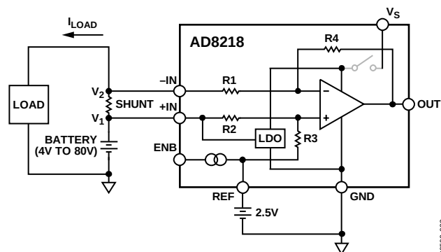
图33. 采用2.5 V基准电压输入的双向操作
