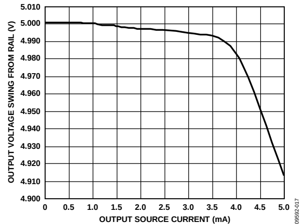
图19. 输出电压摆幅与输出源电流的关系
