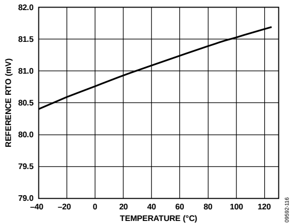
图16. 内部基准电压与温度的关系( V_s = 5\text{ V} , V_s = \text{NC} , V_{CM} = 12\text{ V} , 引脚1(+IN)与引脚8(-IN)短接, 引脚3(ENB)短接至引脚4(GND))
