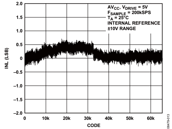
图14. AD7606典型INL, \pm 10V 范围
