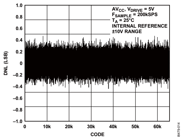
图15. AD7606典型DNL, \pm 10V 范围
