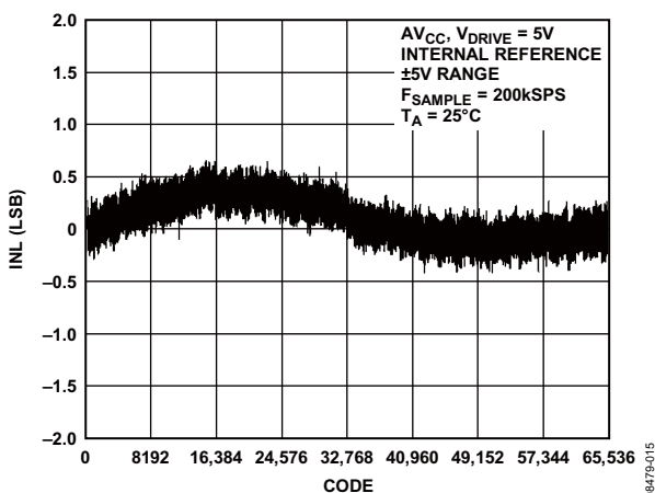
图16. AD7606典型INL, \pm 5V 范围
