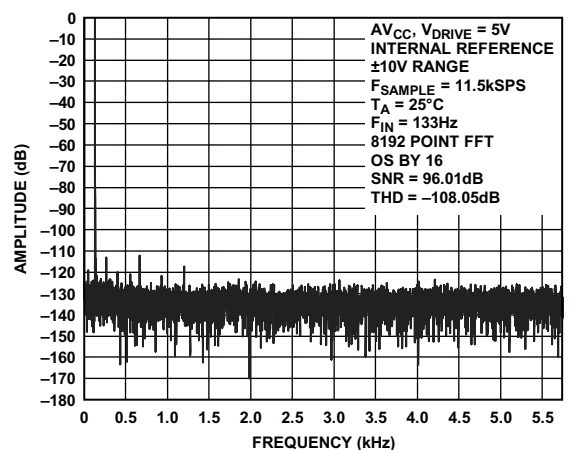
图13. 16倍过采样FFT图, \pm 10V 范围
