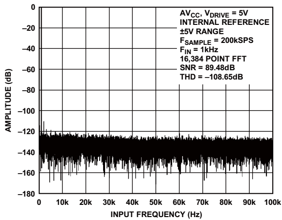
图12. AD7606 FFT图, \pm 5V 范围
