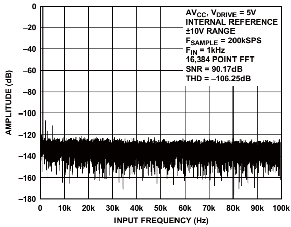
图11. AD7606 FFT, \pm 10V 范围
