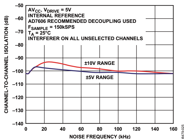
图28. 通道间隔离
