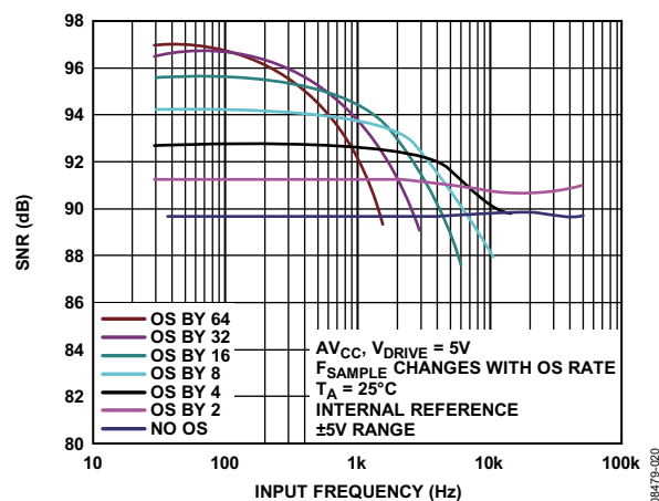
图26. 不同过采样率下SNR与输入频率的关系, ±5 V范围
