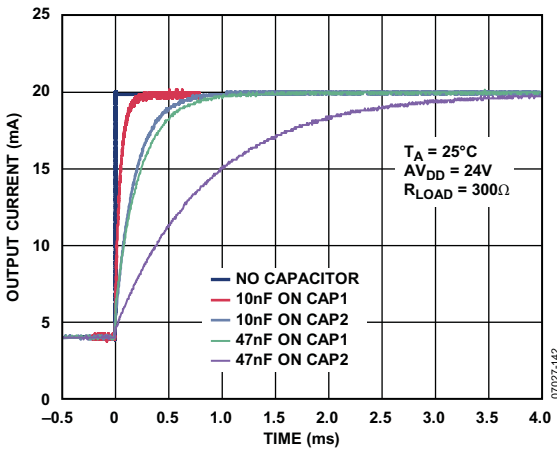
图44. CAP1和CAP2引脚上连接外部电容时，压摆控制的4 mA至20 mA输出电流步进变化
