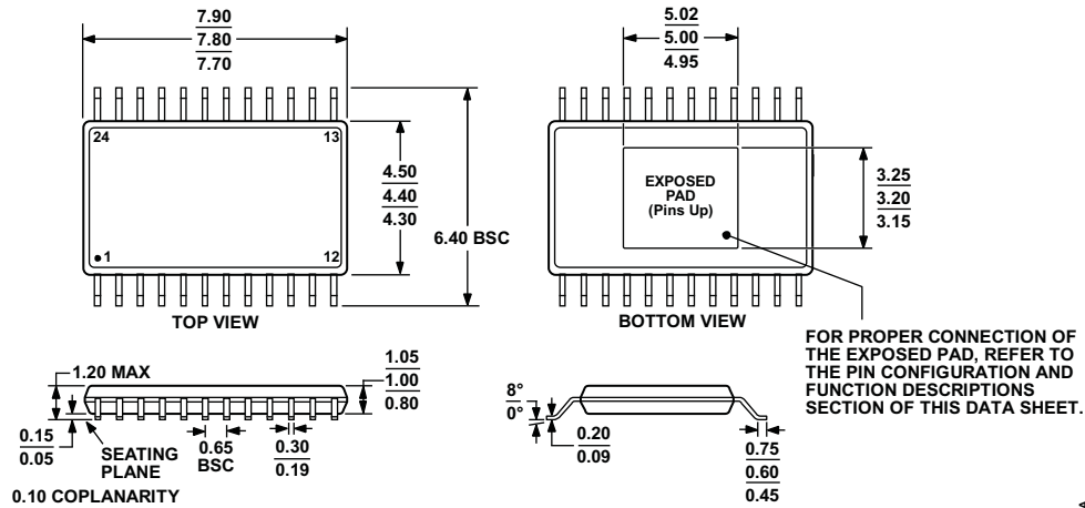
图54. 24引脚超薄紧凑小型封装、裸露焊盘 [TSSOP_EP] (RE-24)
