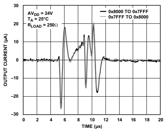
图35. 数模转换毛刺
