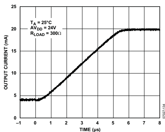
图36. 4 mA至20 mA输出电流步进
