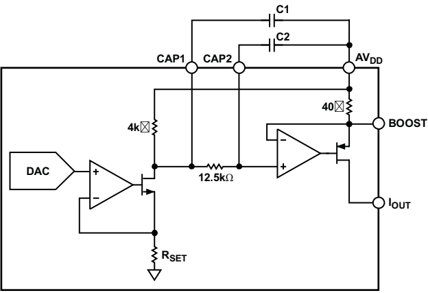
图43. I OUT 滤波电路
