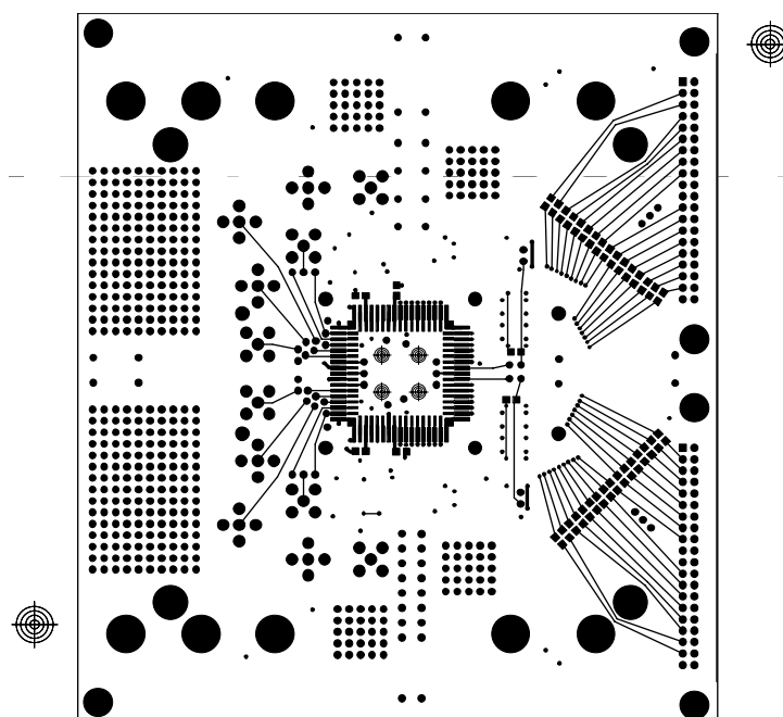
Figure 25. Top Layer
