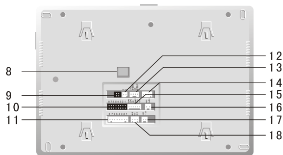
后视图
