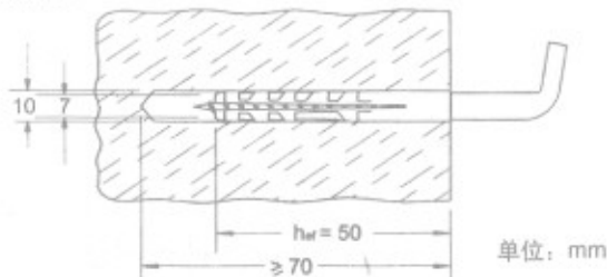
图五 挂钩螺钉的安装
