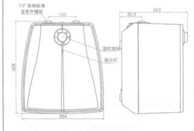
图二 EWH-6B 外观特征
