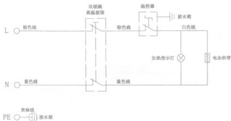
图十 壁挂式电热水器的接线图
