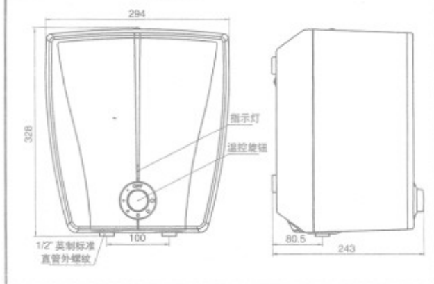
图一 EWH-6 外观特征
