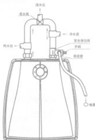
图八 EWH-6B 管道连接图 (示意图)
