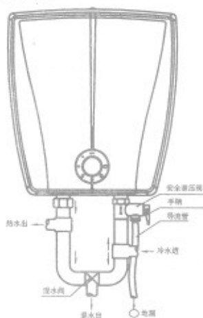
图七 EWH-6 管道连接图 (示意图)
