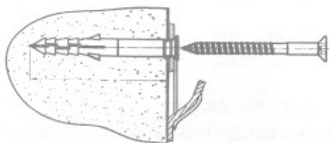
图五 固定挂板的安装
