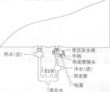
图八 管道连接图
