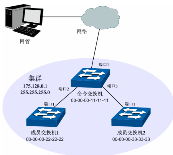
图 13-15 集群管理组网图
