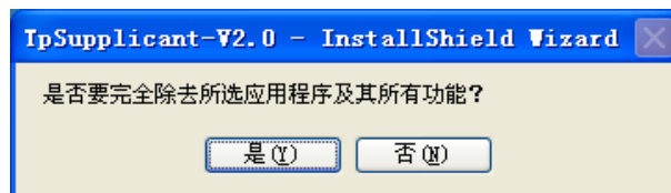
图 9 卸载软件
