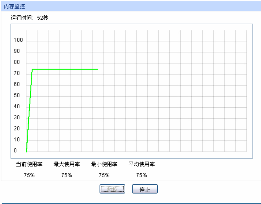
图 14-2 内存监控
