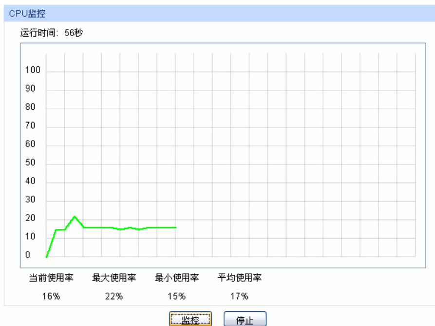
图 14-1 CPU 监控
