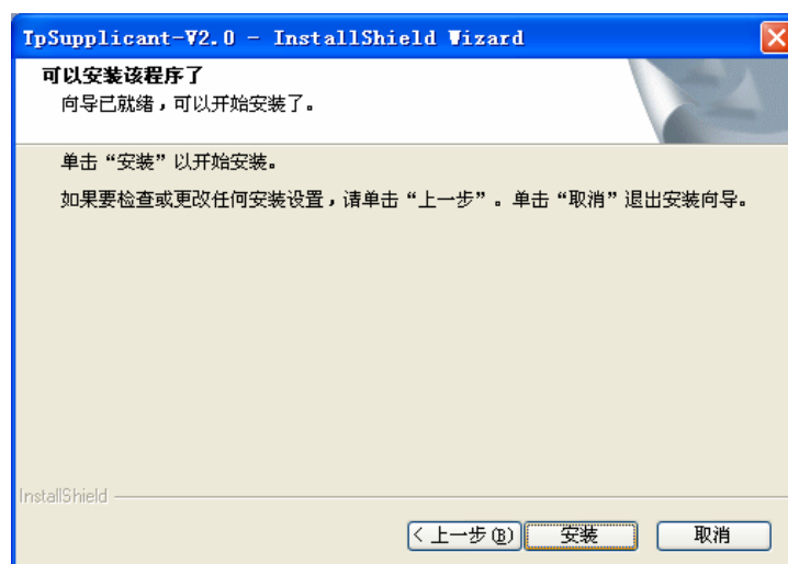
图 5 正在安装
