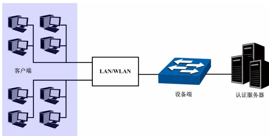
图 11-17 802.1X 认证的体系结构
