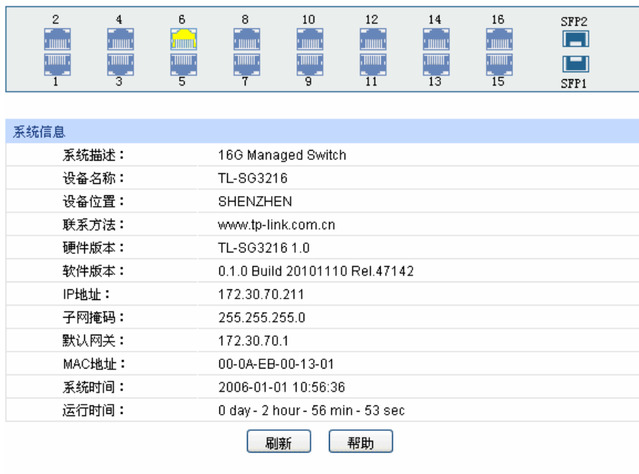
图 3-2 系统信息
