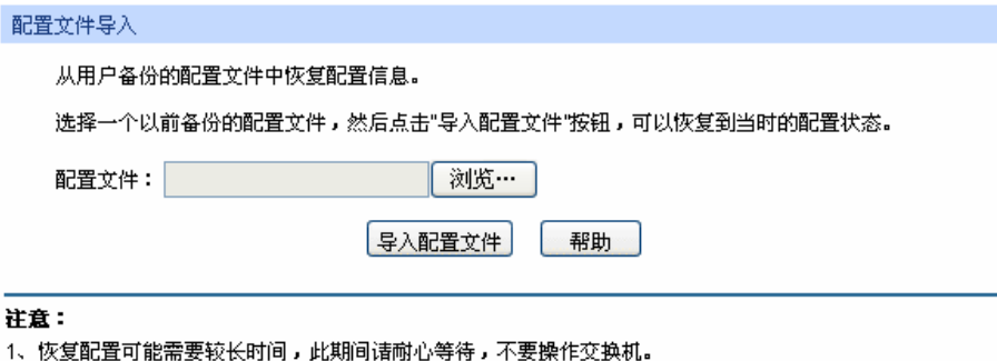
图 4-9 配置导入
