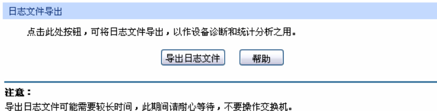
图 14-6 日志导出
