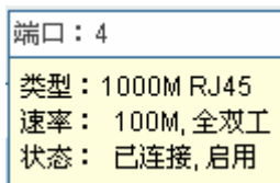
图 4-2 端口信息
