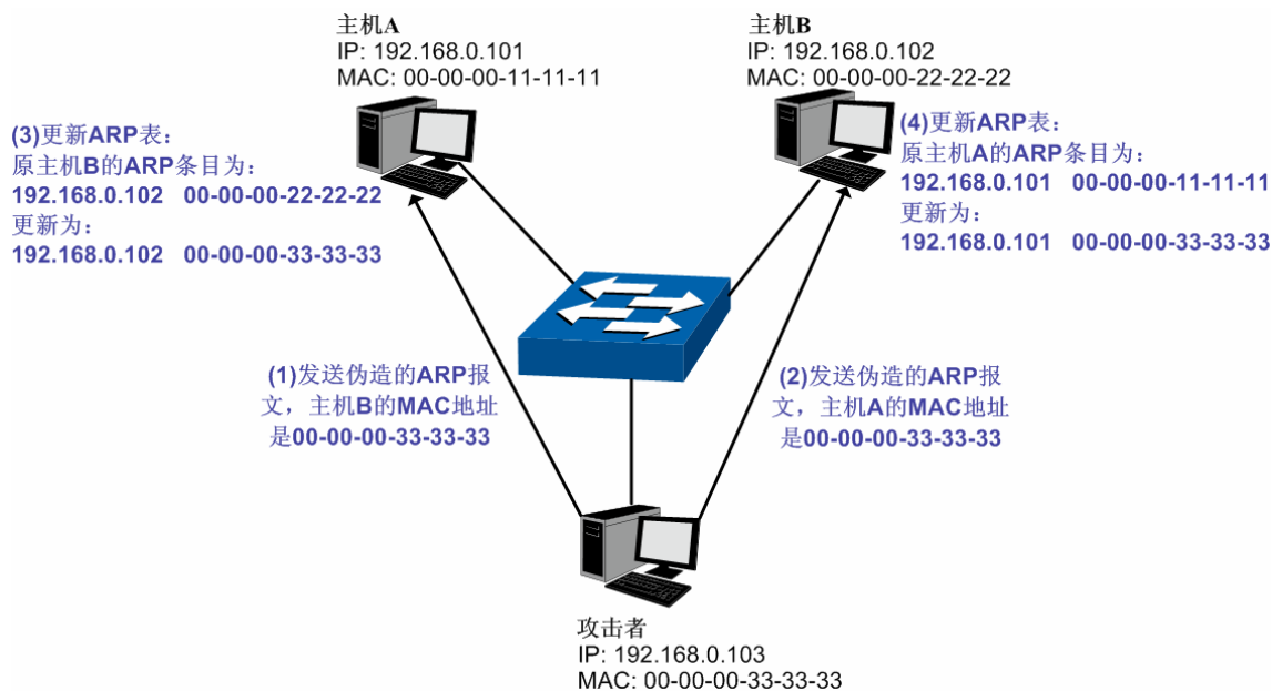
图 11-12 中间人攻击
