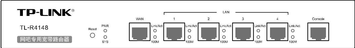
图 3.1 前面板示意图
