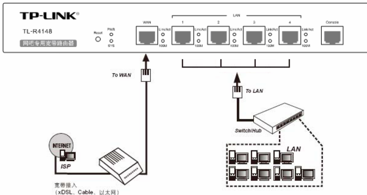
图 3.7 建立局域网和广域网连接
