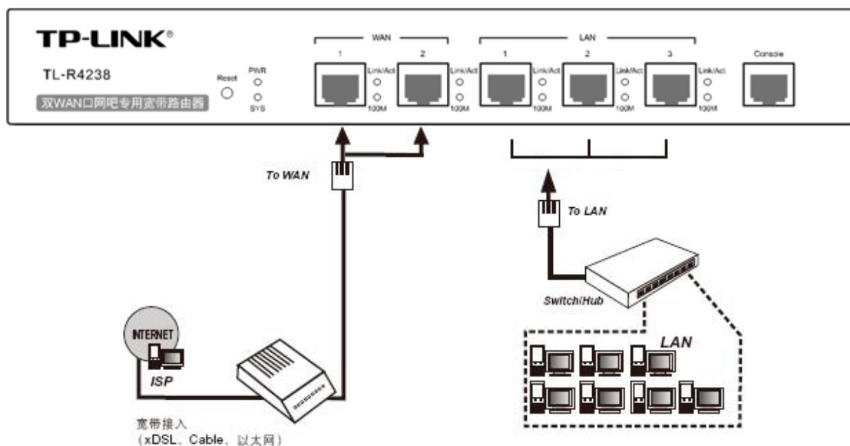
图 3.7 建立局域网和广域网连接
