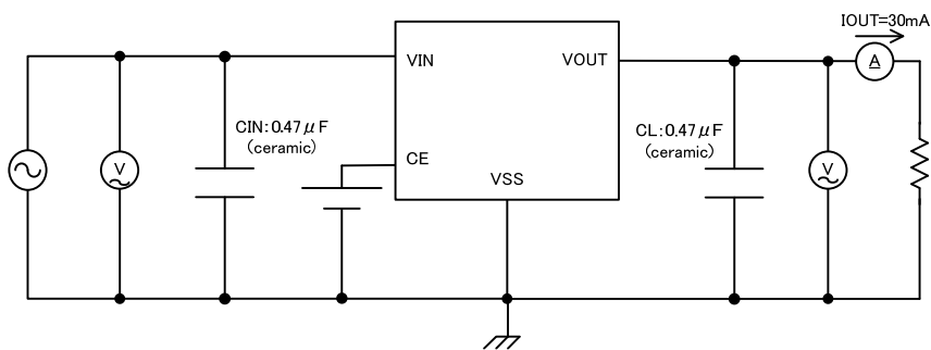
●Circuit ④
