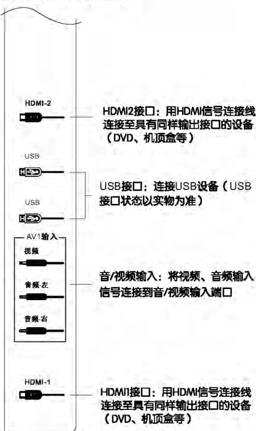
侧AV端子右示意图
