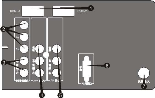
后AV端子示意图
