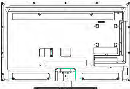
背面示意图
