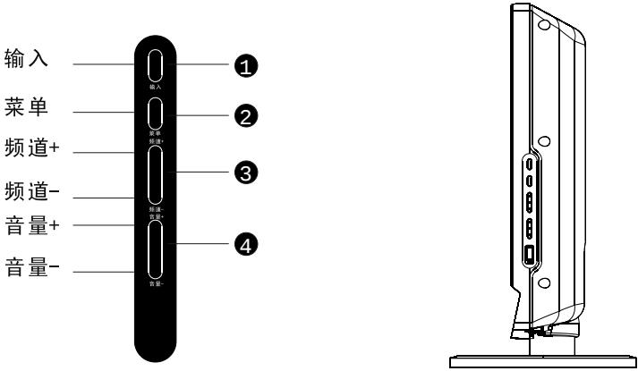
侧面按键示意图
