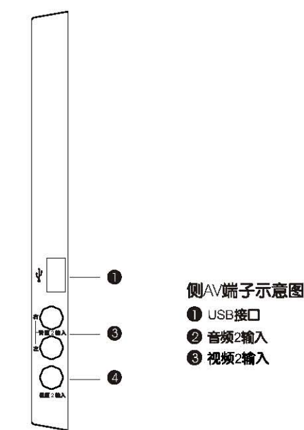
侧AV端子示意图
