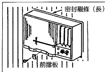
圖6 使用“密封襯條”(長)(附件)，予以密封(剪切至所需長度)嵌進牆壁與機殼之間，裝上“前擋板”。
