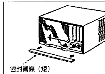
圖5 將底盤推入“機殼”後將“密封襯條”(短)(附件)擠入“底盤”和“機殼”的中間。
