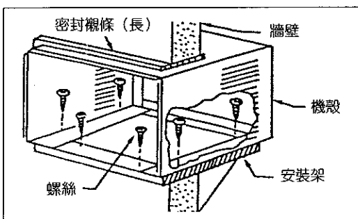
圖4 用固定螺絲固定機殼於安裝架上。
