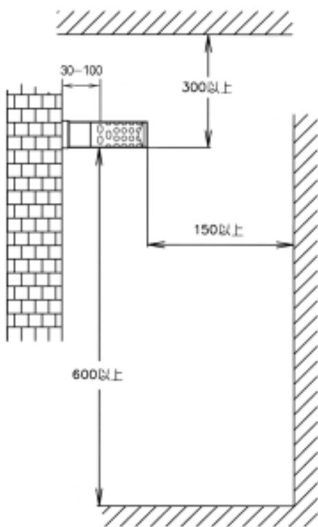
排气管出口侧面
