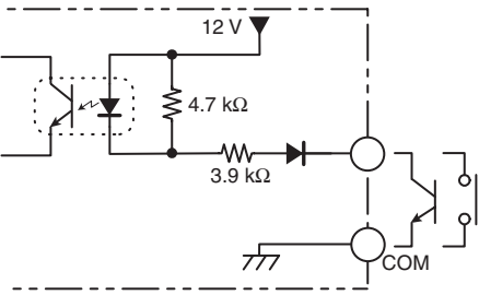
< 电路图 >
