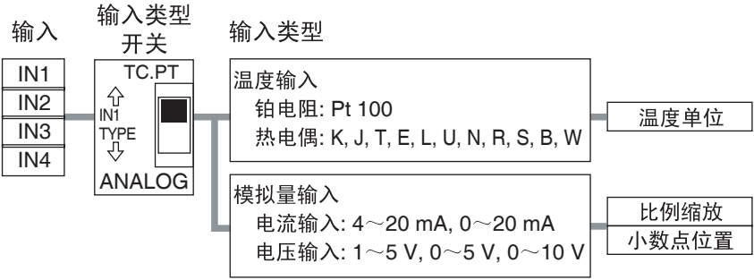
输入类型开关位置
