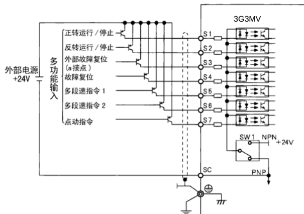
PNP 晶体管顺控器的接线图 (24V 公共点)
