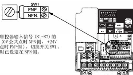
NPN 晶体管顺控器的接线图 (0V 公共点)
