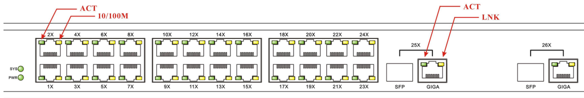
图 2.5 Netcore 7224NSM LED 指示灯示意图片
