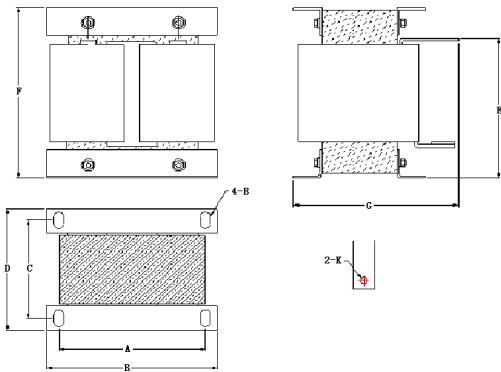
图2-10外置电抗器尺寸示意图
