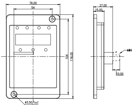
图2-8 外引键盘外型尺寸示意图
