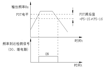
图6-18 FDT电平检测示意图
