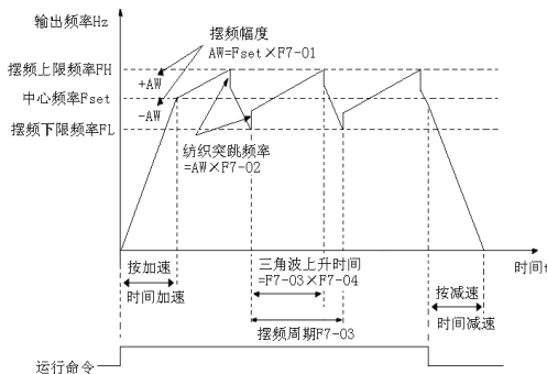
图6-22 摆频运行示意图
