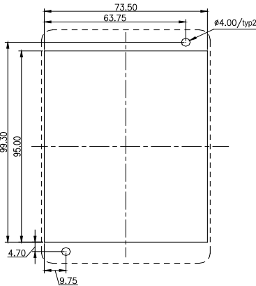
图2-9 外引键盘安装开孔示意图
