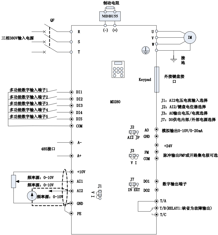
图3-6 MD280T37G/45P~MD280T55G/75P三相变频器接线示意图
