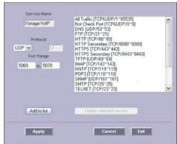
Add Vonage VoIP Service
