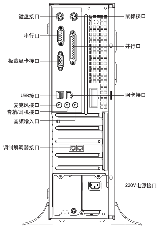
后面板图示 1
