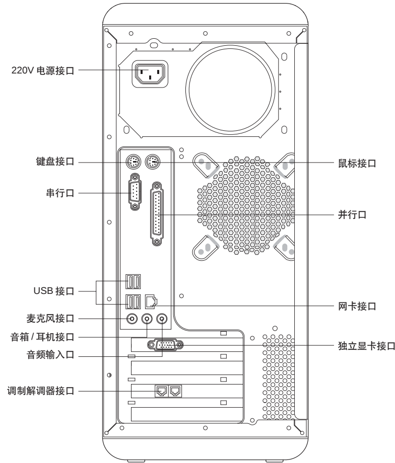
后面板图示 1
