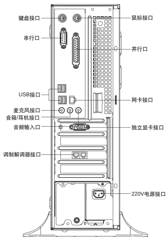
后面板图示 2
