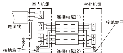
图14 室内外电气连接图
