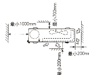
图4 机器户外部分所需空间
