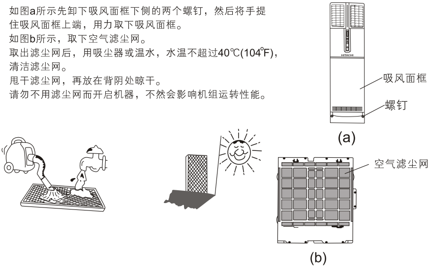
空气滤尘网的拆卸示意图
