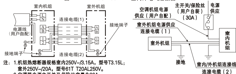
图14-2 RAP/C-L53AVX 室内外电气连接图
