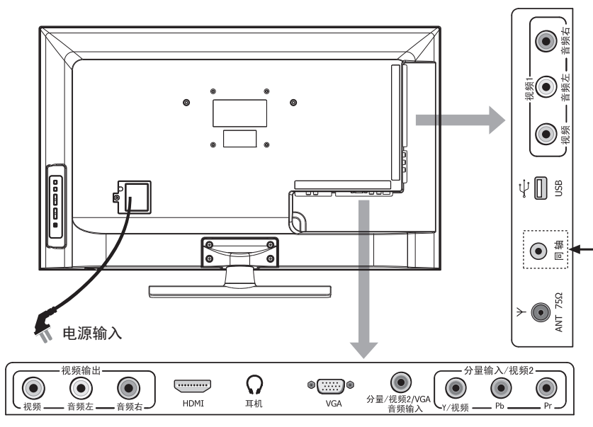
后视图
