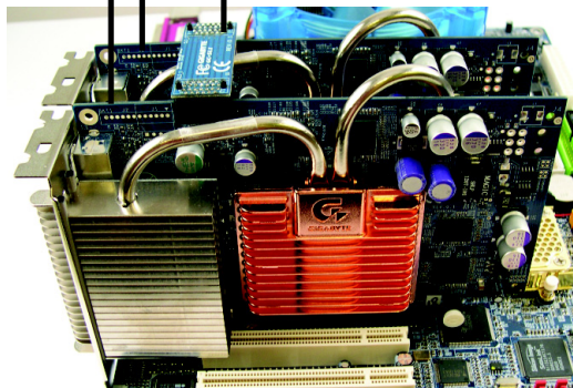
兩張相同型號的顯示卡 (例：GV-NX66T256DP-RH) SLI 連結器 (由主機板廠商提供)
