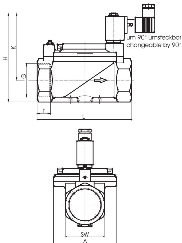
Maßzeichnung Standardausführung Dimensional drawing of standard type
