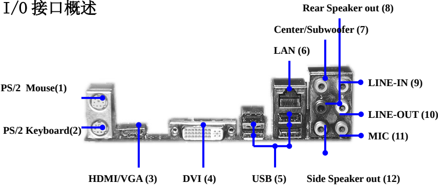
I/O 接口部件一览表
