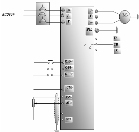
图 4-3 接线示意图 3
