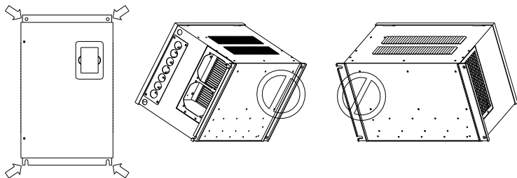
图 1-6 变频器安装示意图
