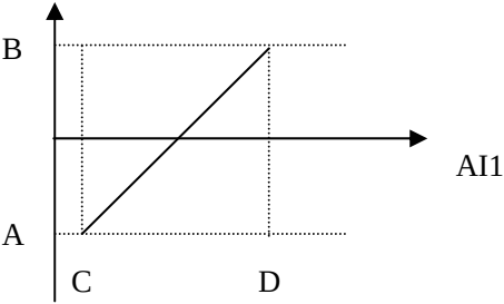
图 5-7 模拟给定与设定量的计算关系
