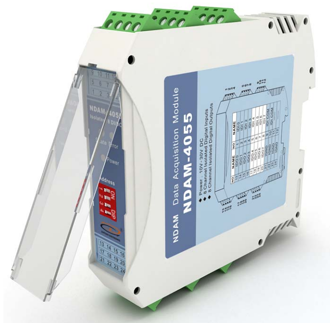
图 2.1 NDAM-4055 外观
