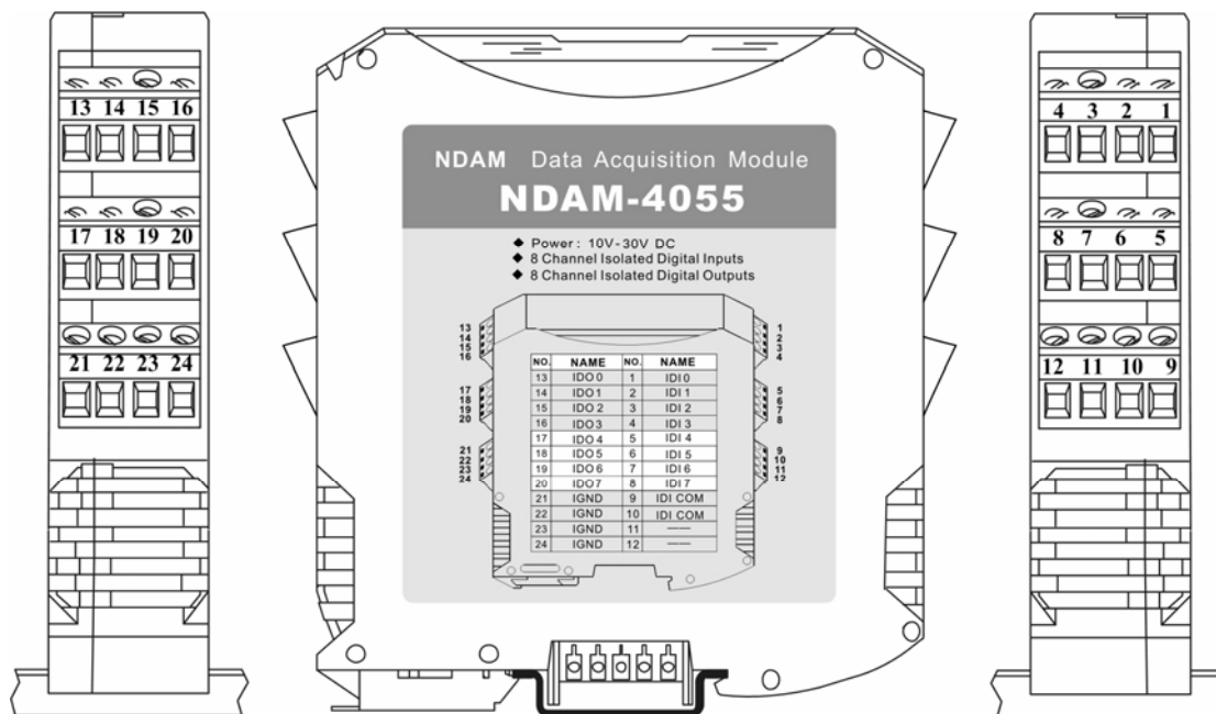
图 2.3 端子排列
