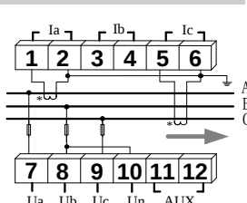
三相三线
