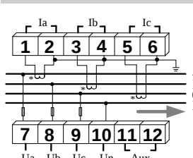
三相四线
