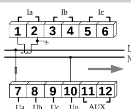
三相四线平衡/一相两线
