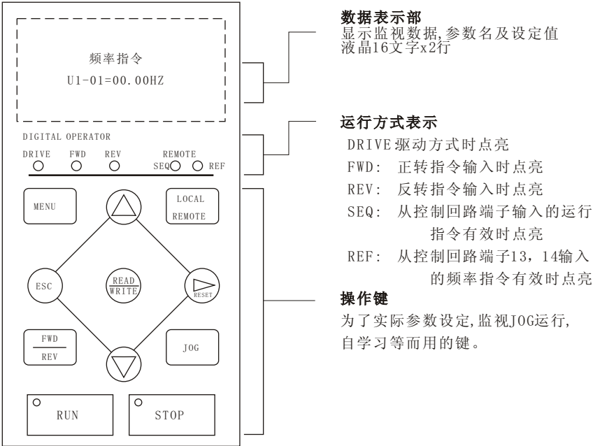
数字操作器(操作器)的各部名称和功能 操作键的功能
