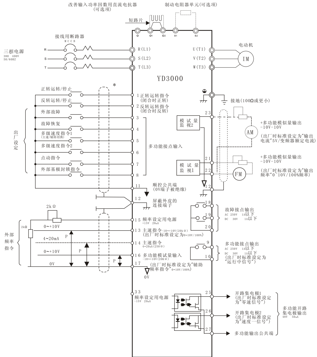
连接图(以YD37P5为例)
