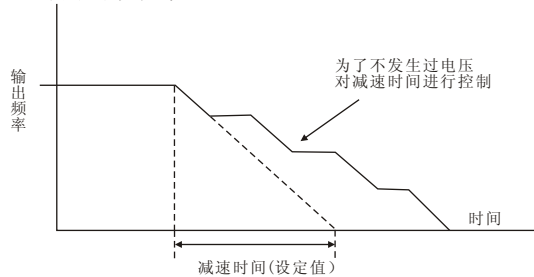
减速中失速防止动作 (L3-04=1 的场合)
