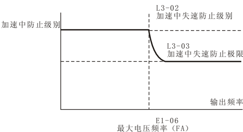
加速中失速防止极限
