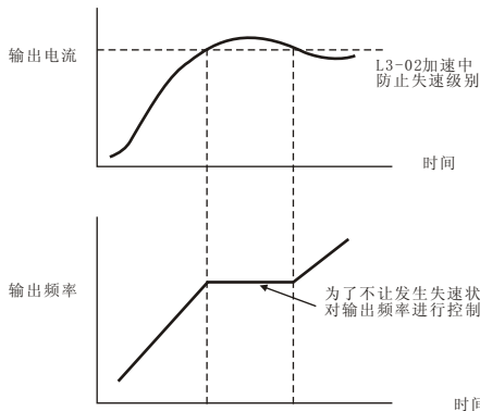
加速中失速防止功能 (L3-01=1的场合)
