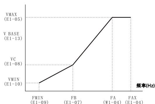
任意V/f曲线
