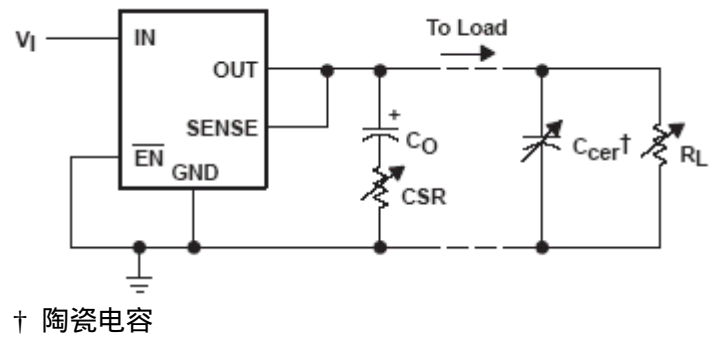
图 6 典型稳定区域的测试电路（参照图 29 至图 32）
