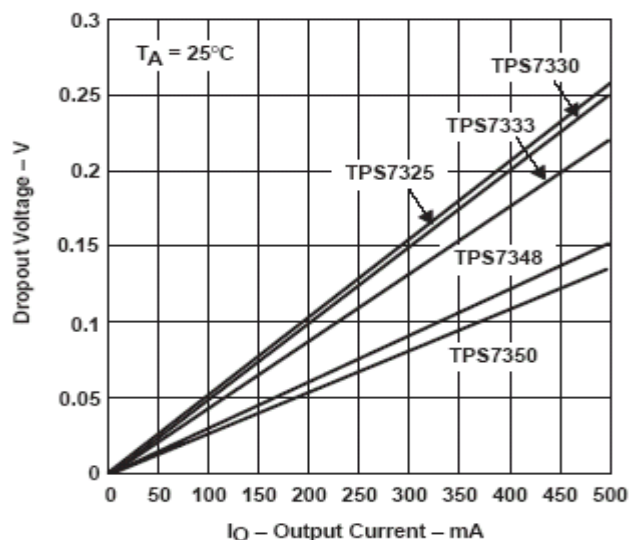
图 1 下降电压与输出电流的关系
