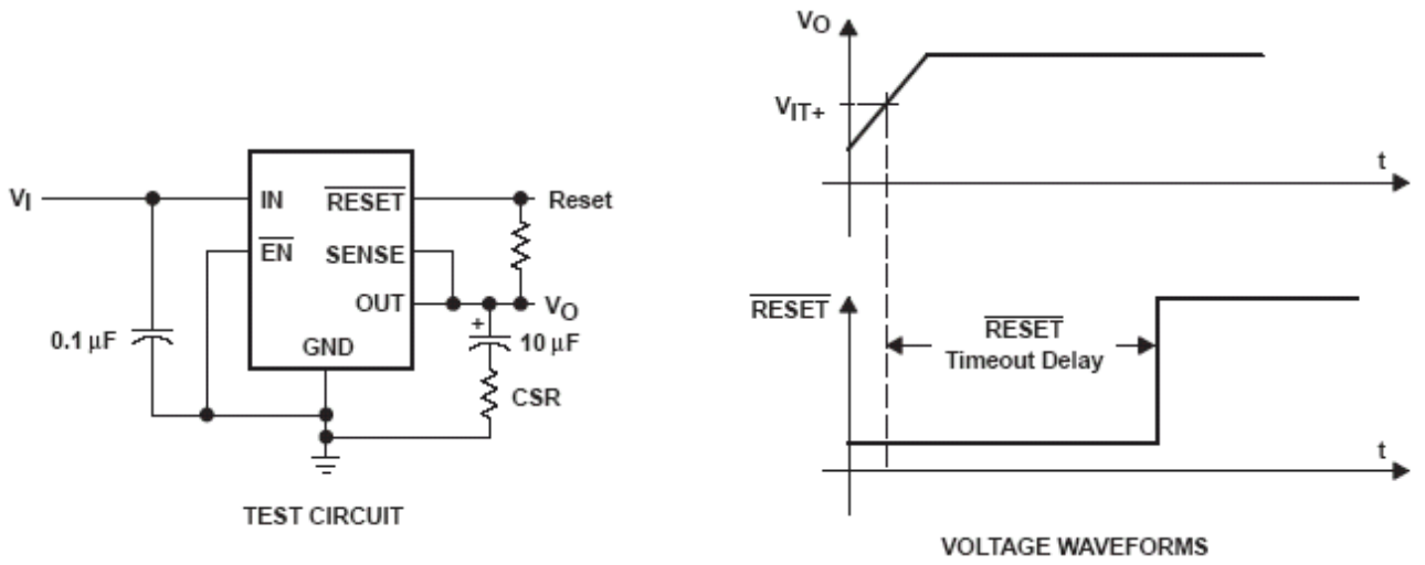
图 5 测试电路与电压波形
