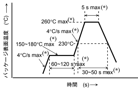
Pb フリーはんだ時の温度プロファイル例
