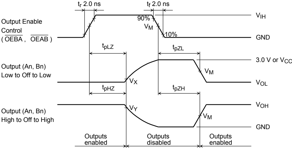
図 6 t_{pLZ} , t_{pHZ} , t_{pZL} , t_{pZH}
