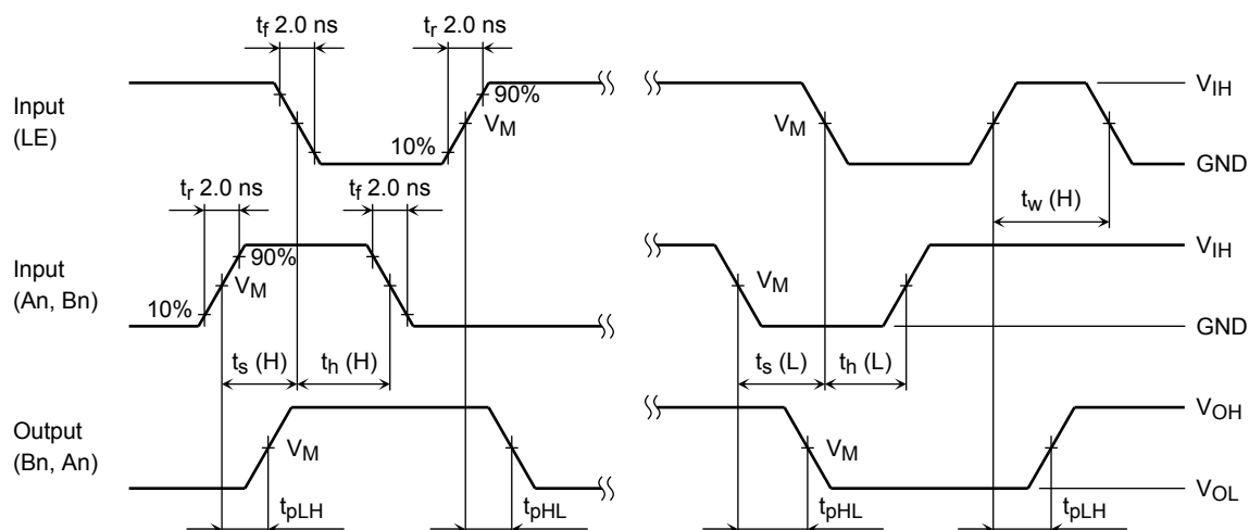
図 4 t_{pLH} , t_{pHL} , t_w , t_s , t_h
