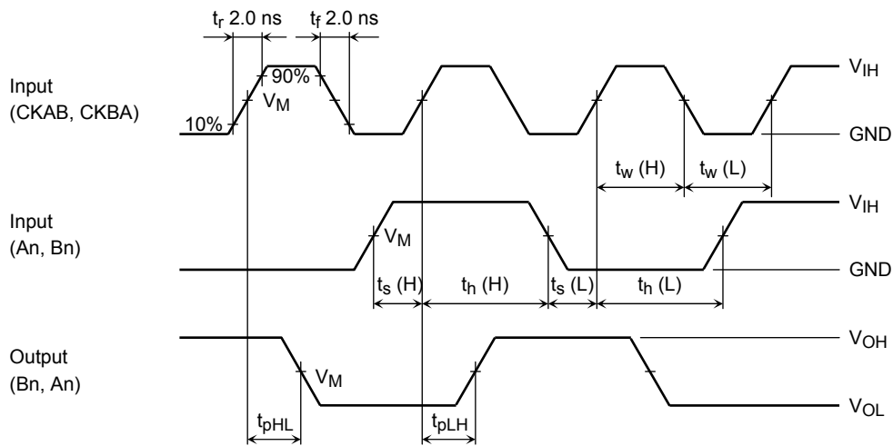
図 3 t_{pLH} , t_{pHL} , t_w , t_s , t_h
