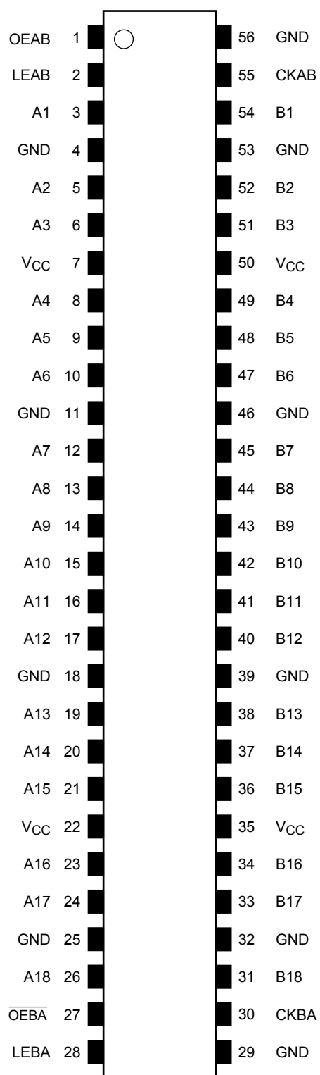
ピン接続図 (top view)
