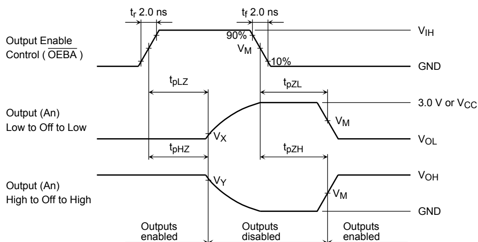
図 5 t_{pLZ} , t_{pHZ} , t_{pZL} , t_{pZH}
