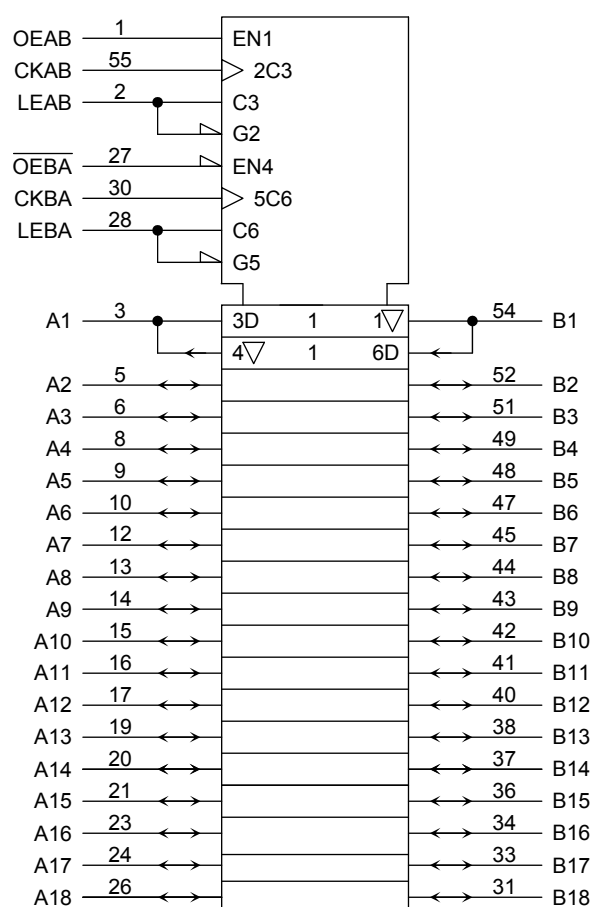
論理図
