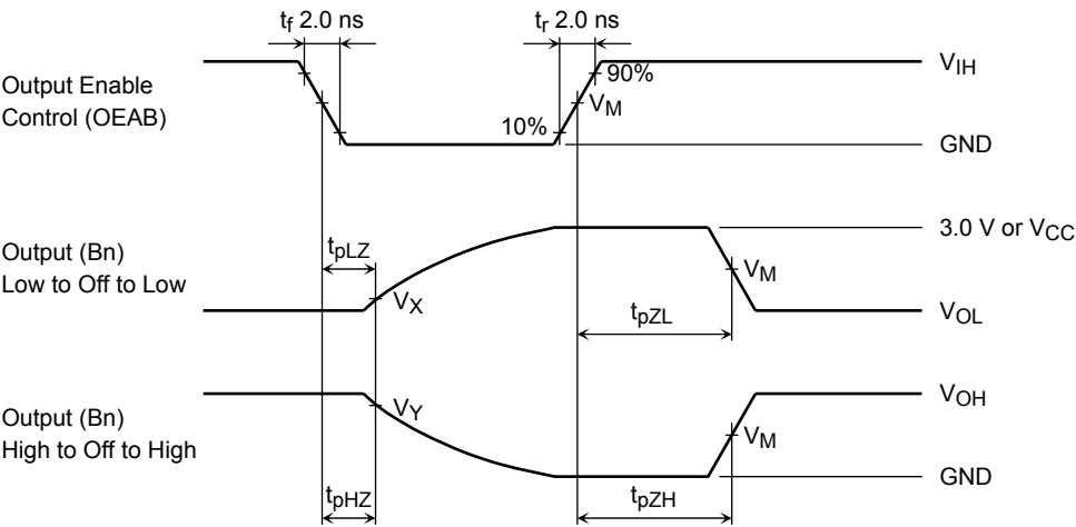
図 6 t_{pLZ} , t_{pHZ} , t_{pZL} , t_{pZH}
