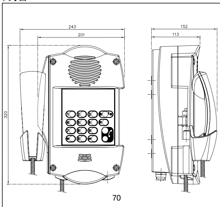
尺寸图
