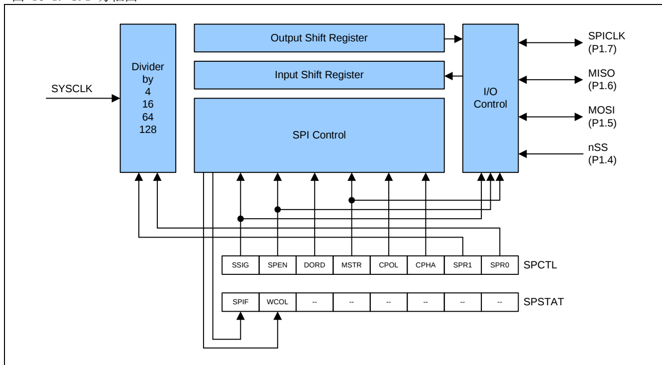
图 15-1. SPI 方框图
