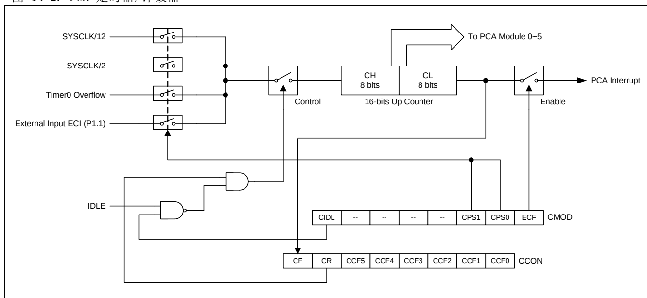
图 14-2. PCA 定时器/计数器
