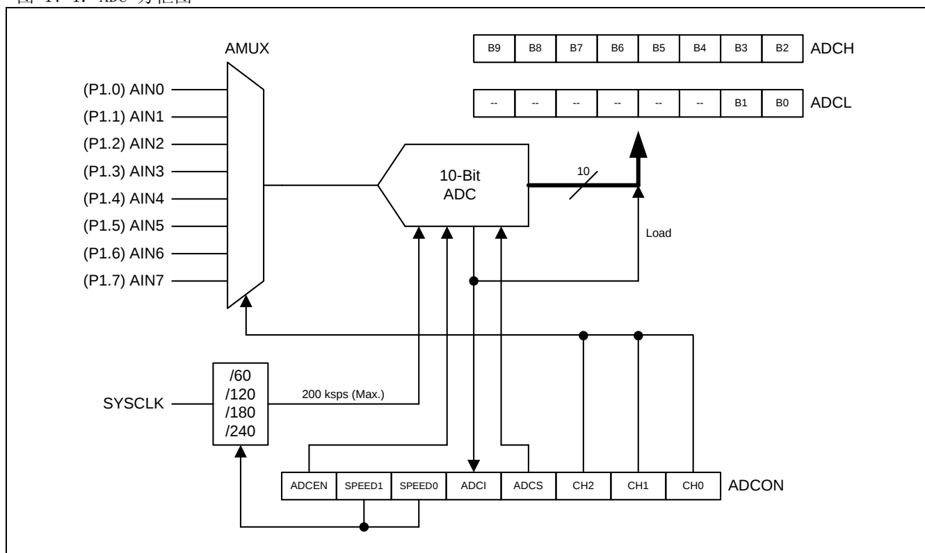
图 17-1. ADC 方框图
