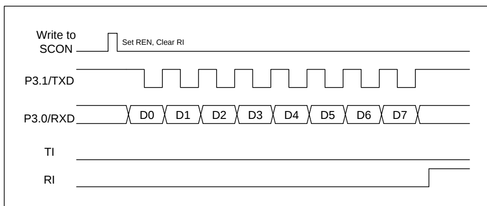
图 12-5 模式 0 接收波形
