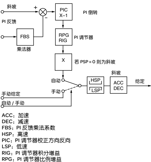
PI 调节器
