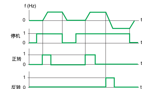
使用 3 线控制的运行举例
