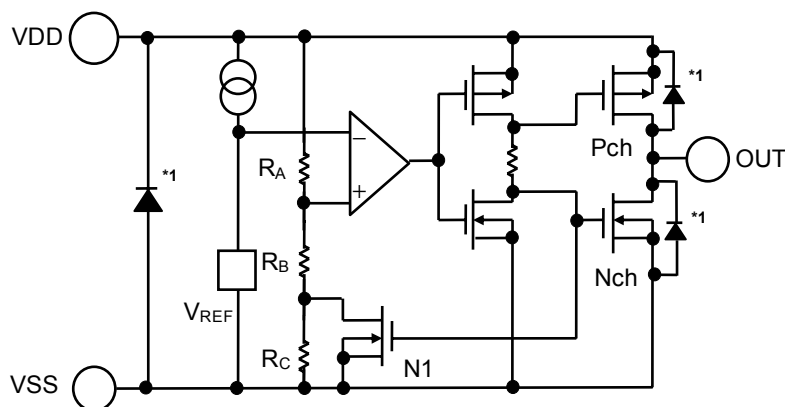
图13 工作说明图1
