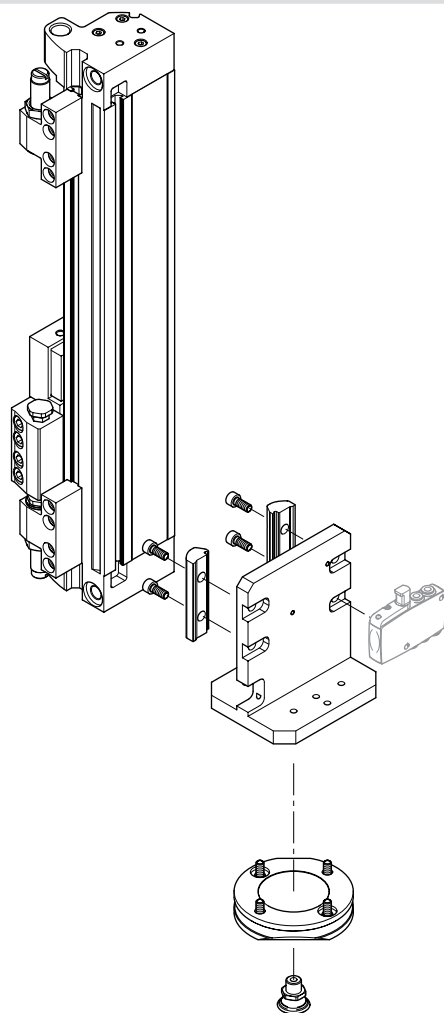
示意图3：RTC系列和SGN系列通过T形转接板和真空转接板进行组合
