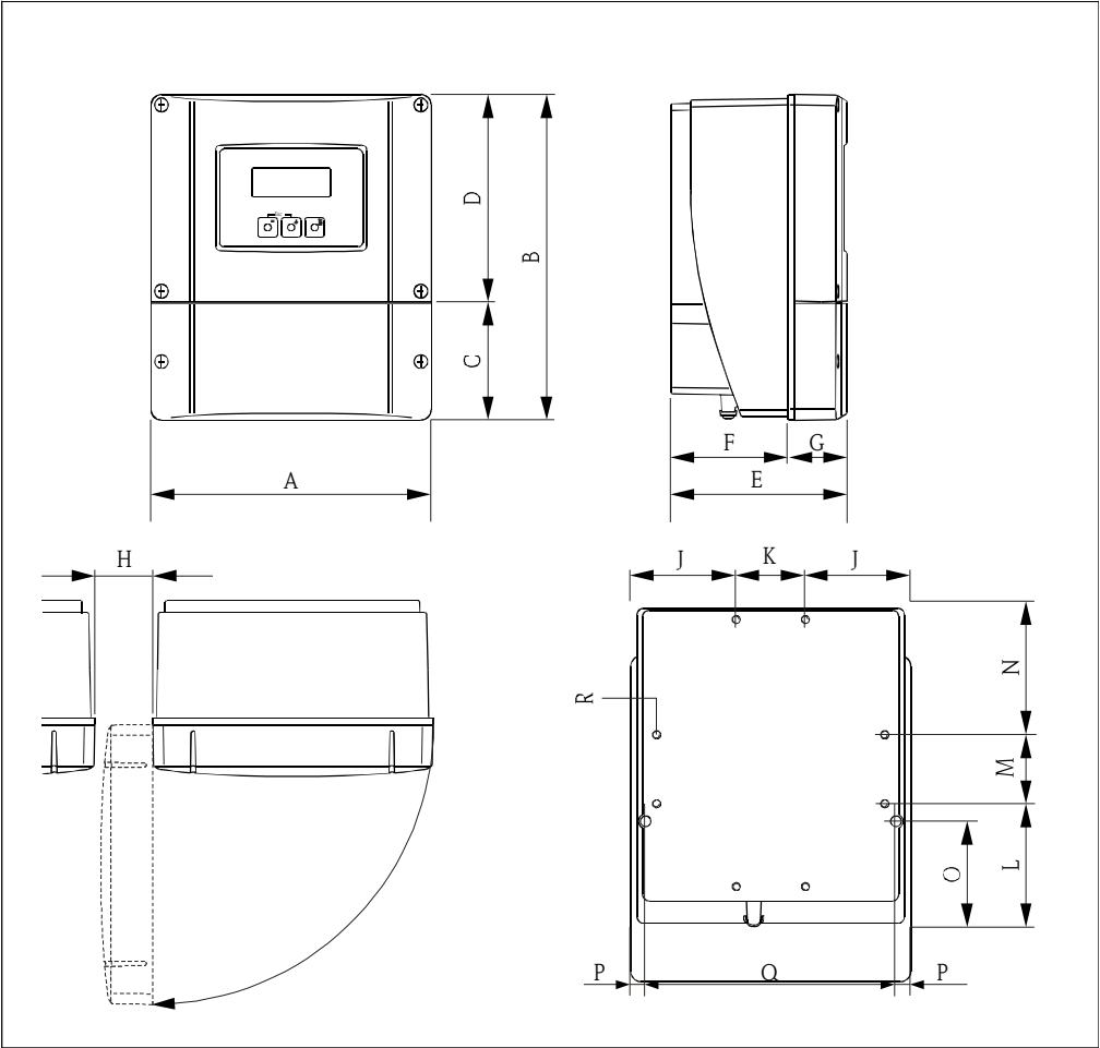
墙装变送器外壳（非防爆区和 II 3G/2 区）
