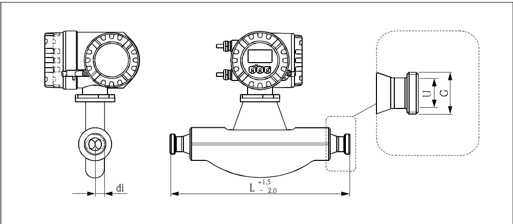
Promass F : DIN 11864-1 Form A 连接 (螺纹接头)
