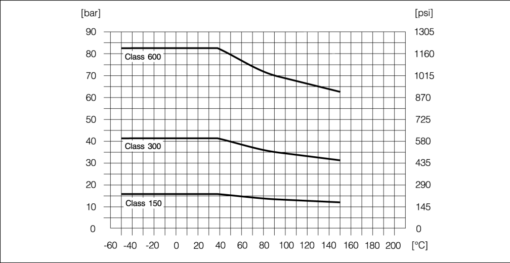
Promass M: ASME B 16.5 法兰连接 法兰材料: 1.4404/316L, 2级钛材
