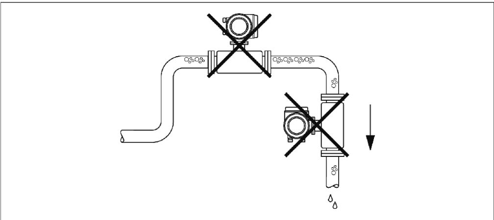
安装位置
