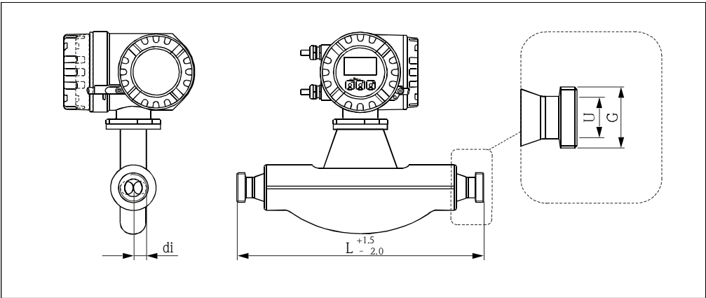
Promass F : DIN 11851 连接 (牛奶接头)
