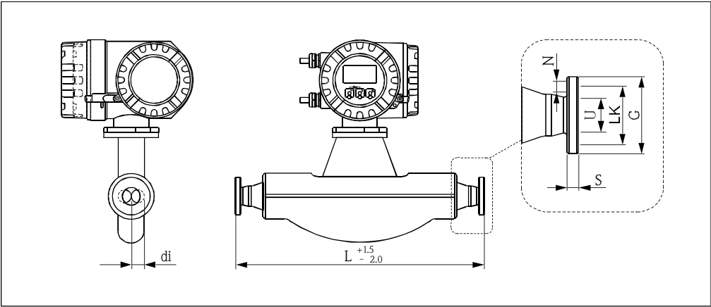
Promass F： DIN 11864-2 Form A 法兰连接（平面法兰）
