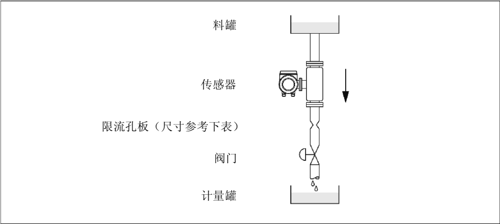
在向下放空管道上安装流量计
