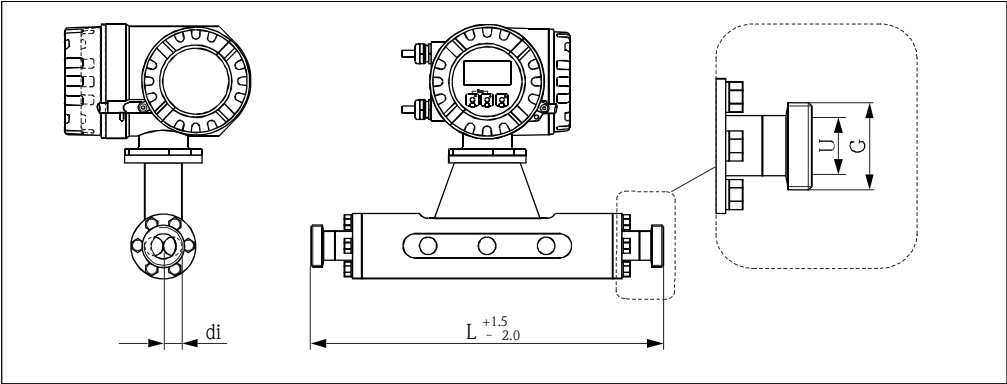
Promass M：DIN 11851 连接（牛奶接头）
