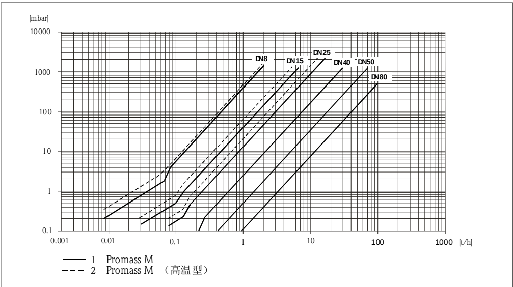
测量水介质的压损图
