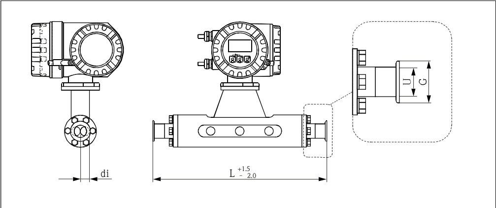
Promass M：三夹头连接
