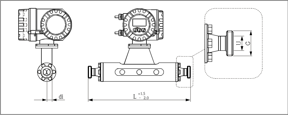
Promass M : DIN 11864-1 Form A 连接 (螺纹接头)
