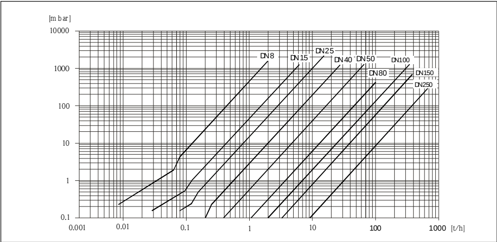
Promass M 的压损系数
