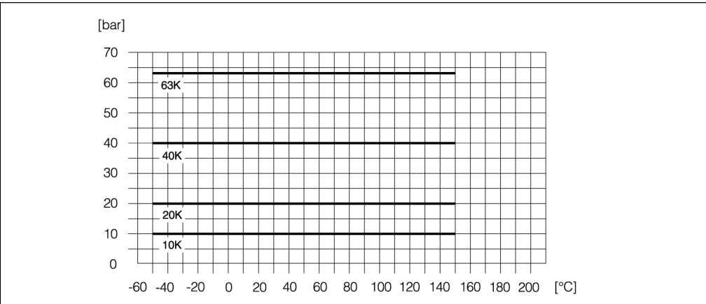
Promass M: JIS B2220 法兰连接 法兰材料: 1.4404/316L, 2级钛材
