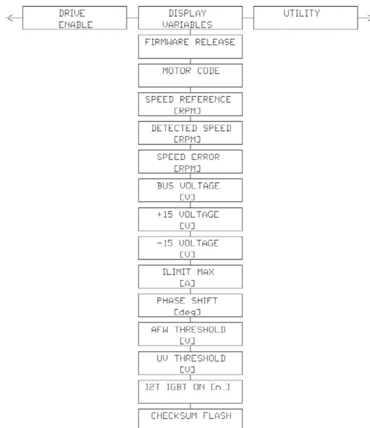
Fig. 6.6 – Display variables menu
