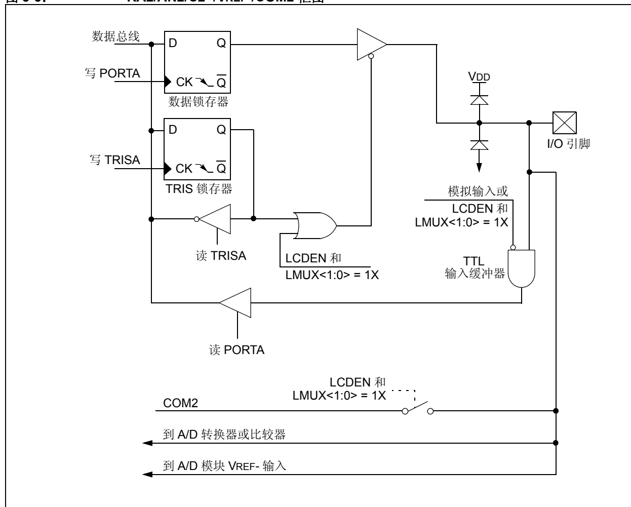
图 3-3: RA2/AN2/C2+/VREF-/COM2 框图
