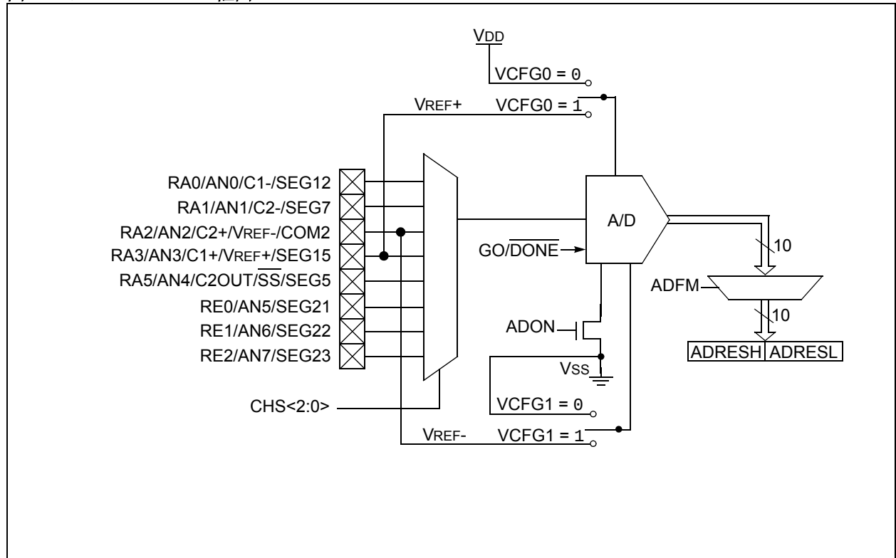
图 12-1: A/D 框图
