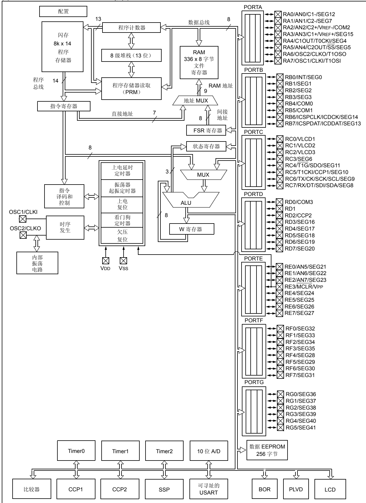
图 1-1: PIC16F946 框图
