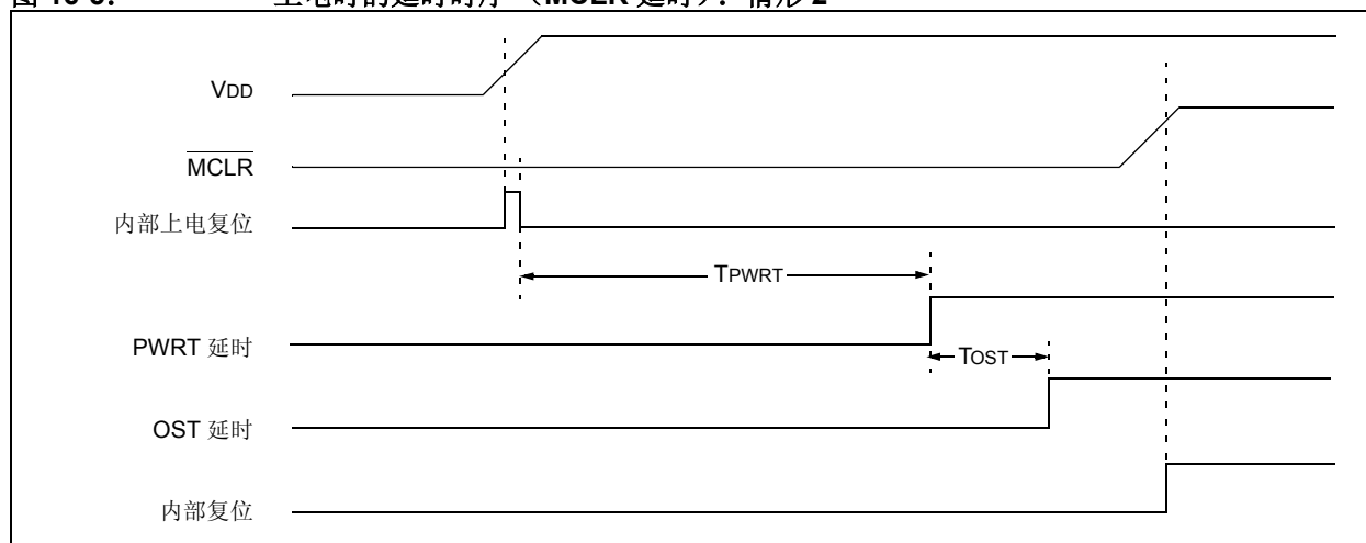
图 16-5: 上电时的延时时序 ( \overline{\text{MCLR}} 延时): 情形 2
