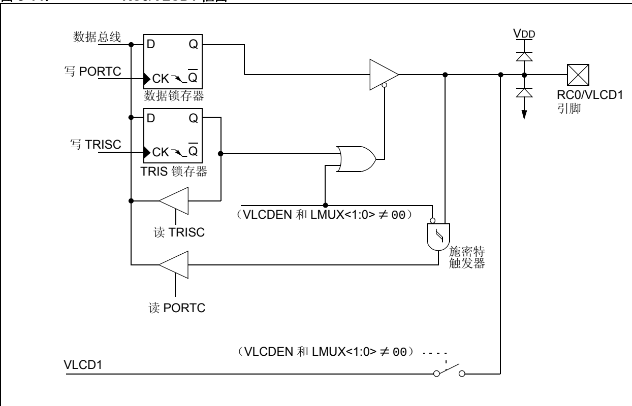
图 3-14: RC0/VLCD1 框图
