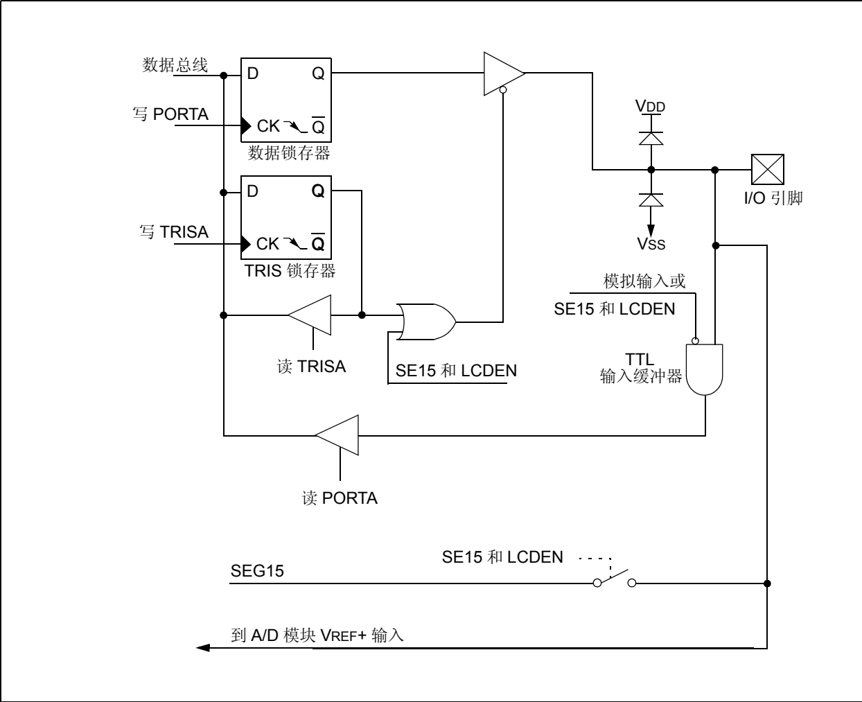
图 3-4: RA3/AN3/C1+/VREF+/SEG15 框图
