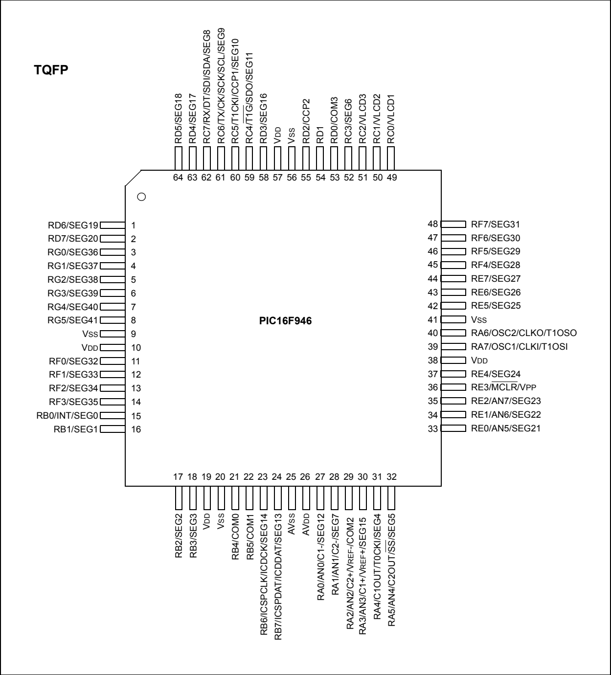
引脚图——PIC16F946
