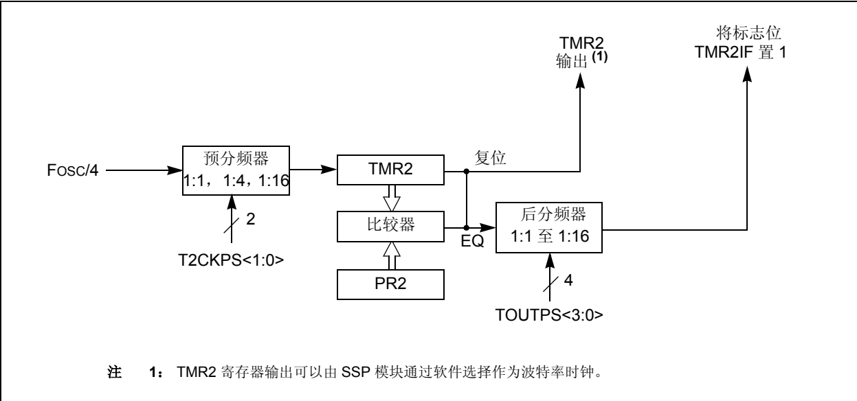
图 7-1: TIMER2 框图
