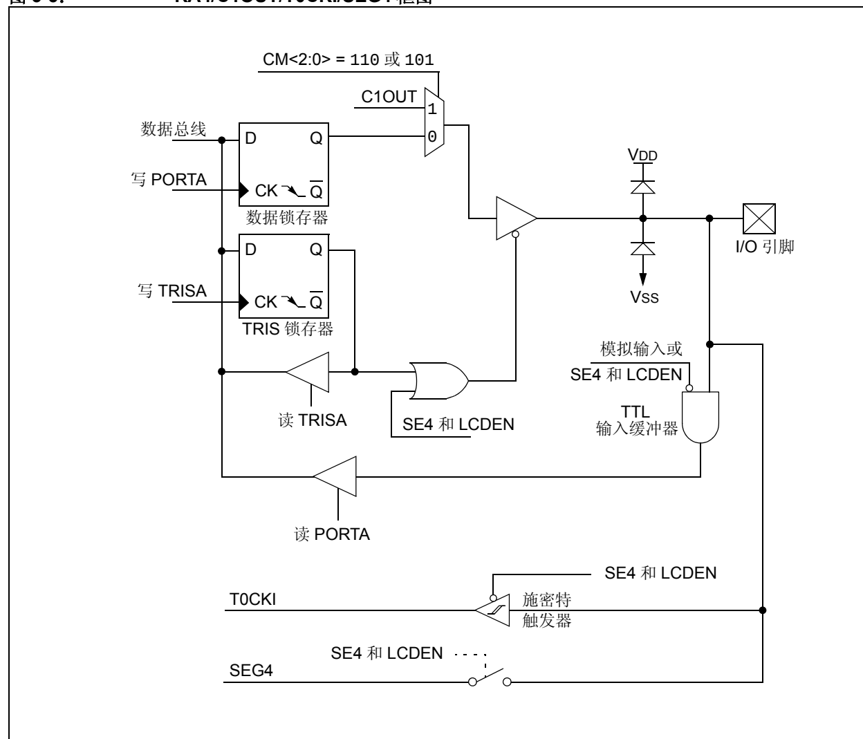
图 3-5: RA4/C1OUT/T0CKI/SEG4 框图
