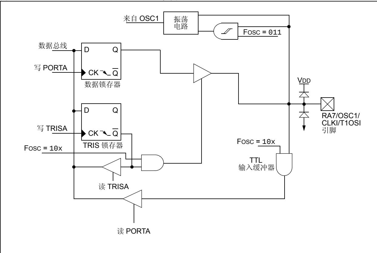
图 3-8: RA7/OSC1/CLKI/T1OSI 框图
