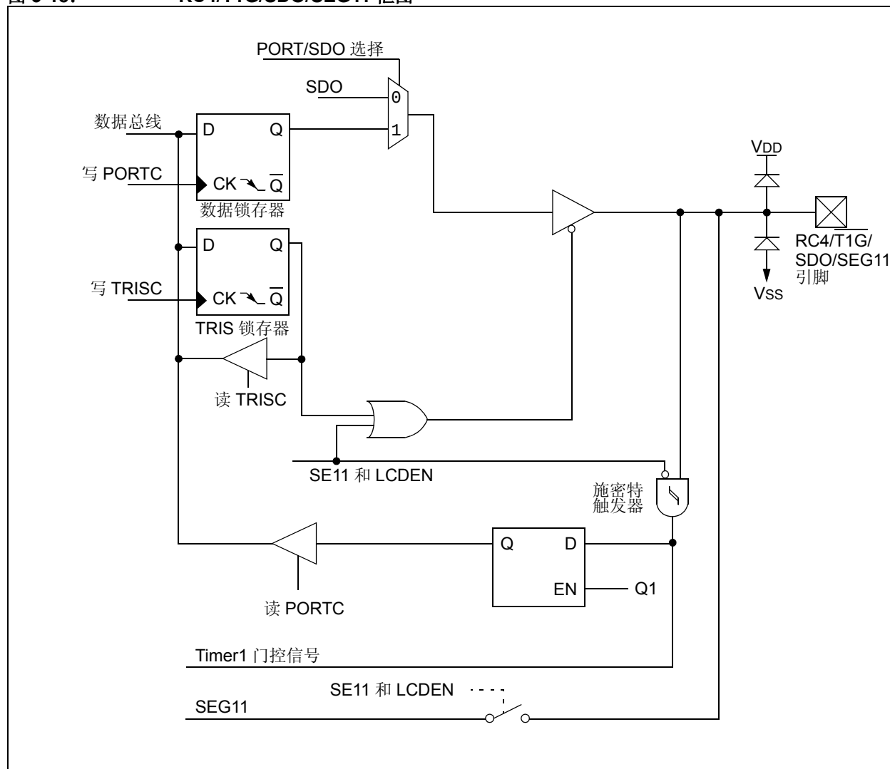
图 3-18: RC4/T1G/SDO/SEG11 框图
