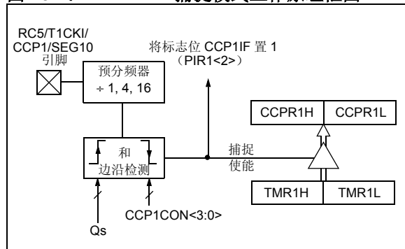
图 15-1: 捕捉模式工作原理框图
