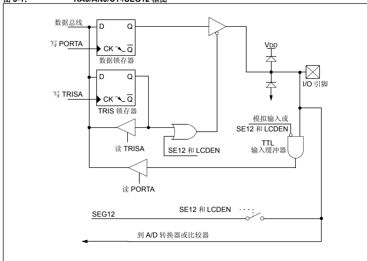
图 3-1: RA0/AN0/C1-/SEG12 框图
