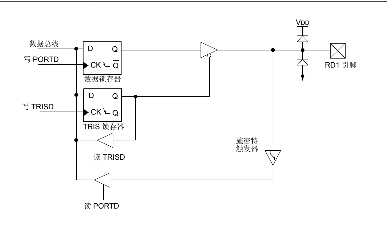
图 3-23: RD1 框图
