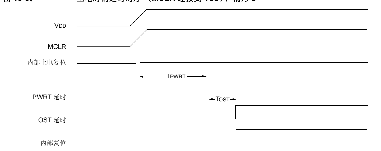
图 16-6: 上电时的延时时序 ( \overline{\text{MCLR}} 连接到 \text{VDD} ): 情形 3
