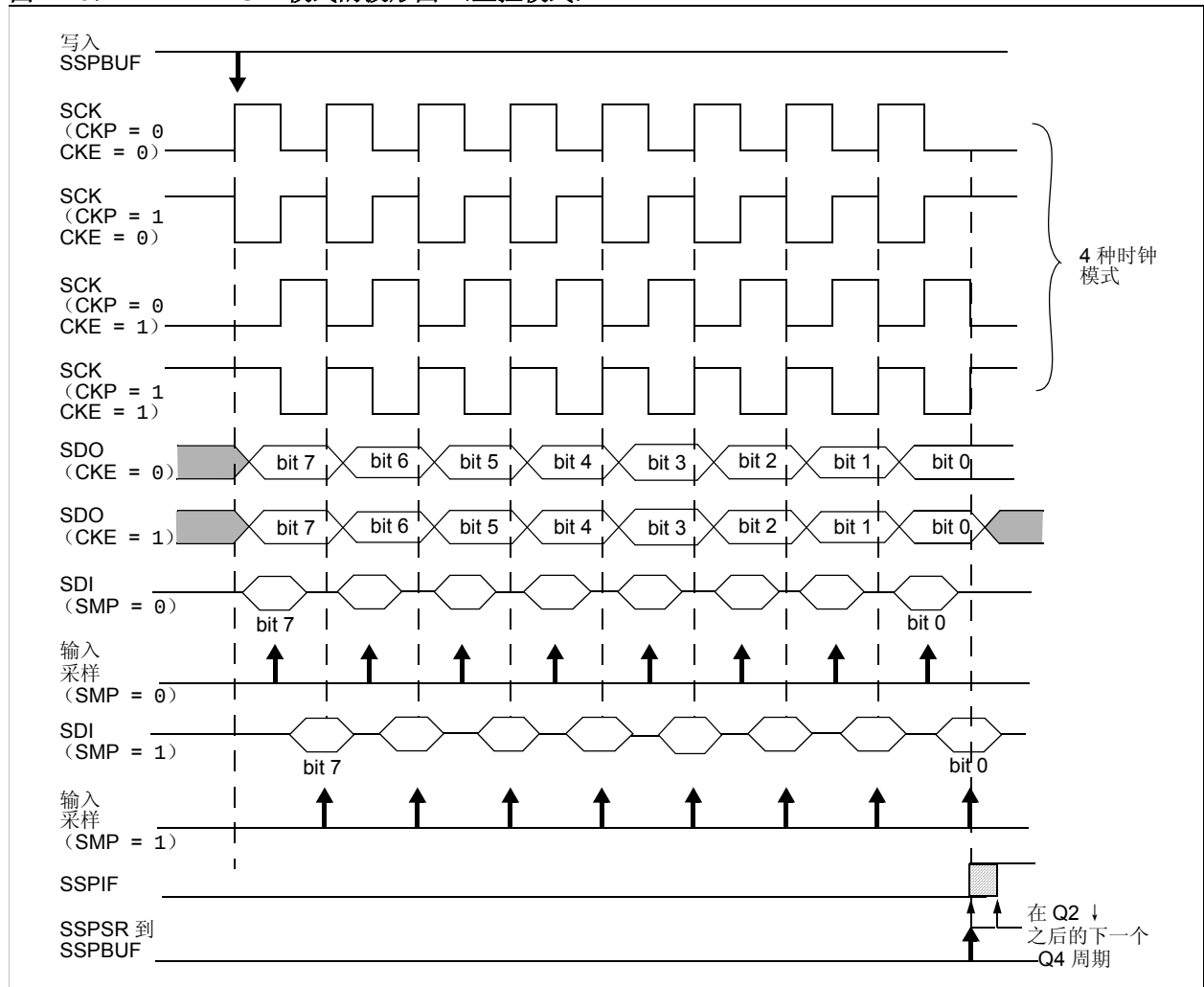
图 14-3: SPI 模式的波形图（主机模式）
