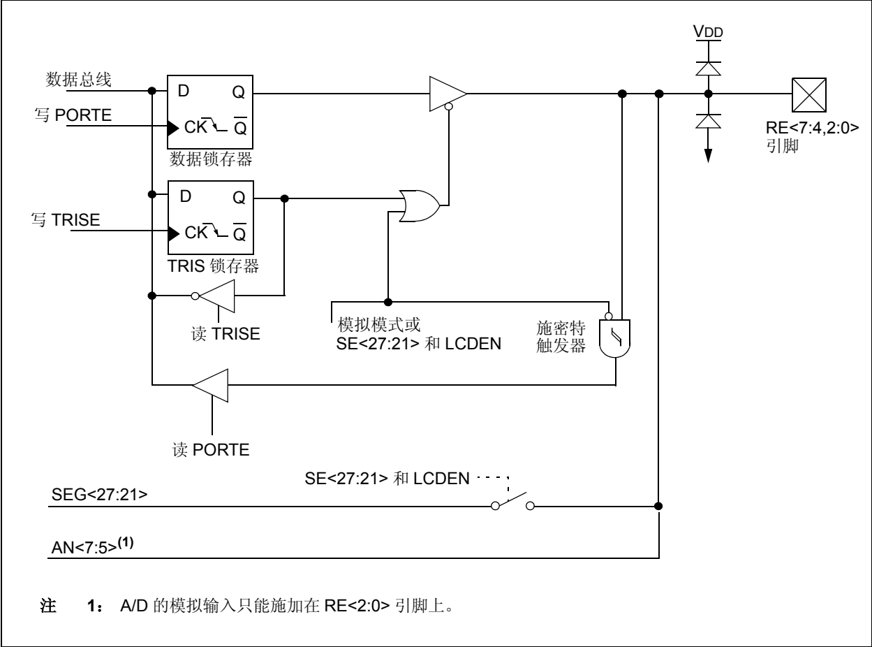
图 3-26: RE<7:4, 2:0> 框图
