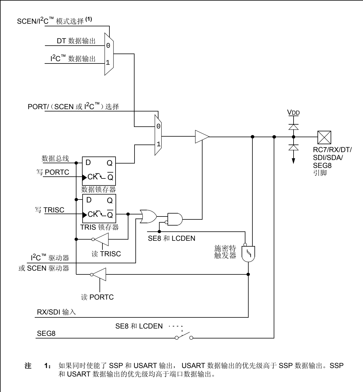
图 3-21: RC7/RX/DT/SDI/SDA/SEG8 框图
