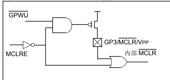
图 8-1: \overline{\text{MCLR}} 选择
