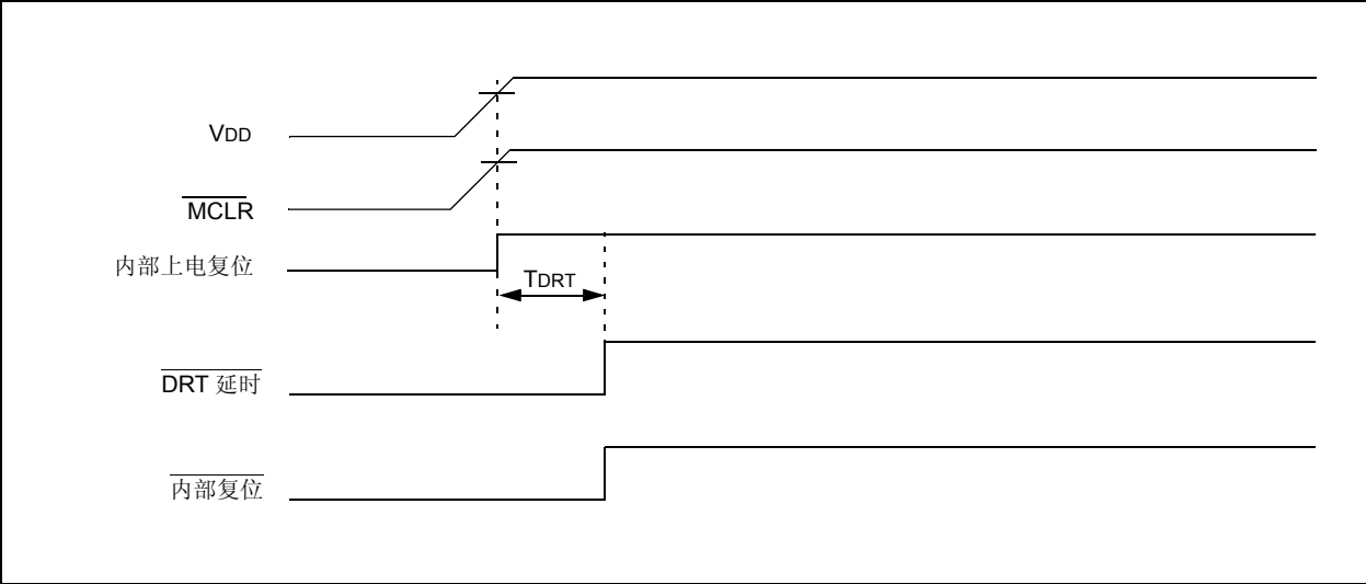
图 8-4: 上电延时时序 ( \overline{MCLR} 连接到 V_{DD} ): 快速 V_{DD} 上升时间
