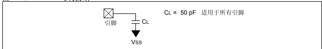
图 10-2: 负载条件
