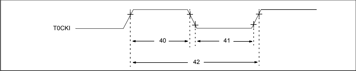
图 10-4: TIMER0 时钟时序
