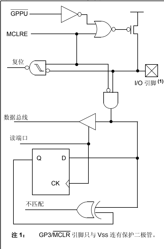
图 5-4: GP3 框图
