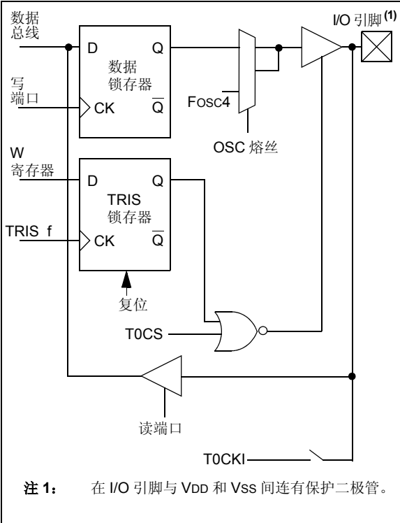
图 5-3: GP2 框图
