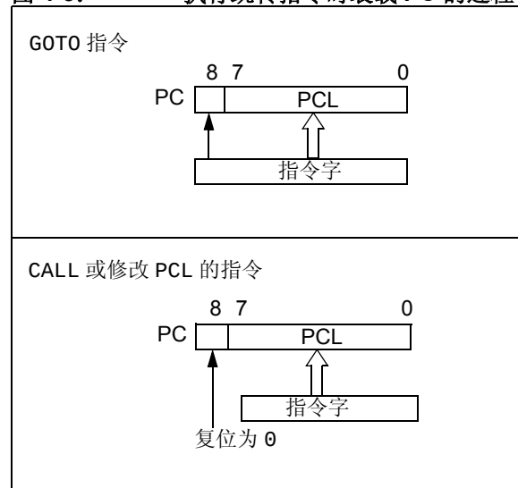
图 4-5: 执行跳转指令时装载 PC 的过程
