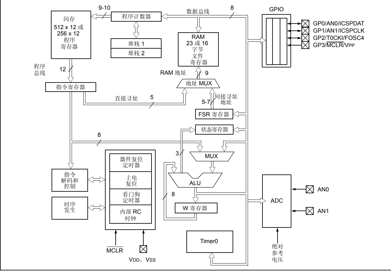
图 3-1: 框图
