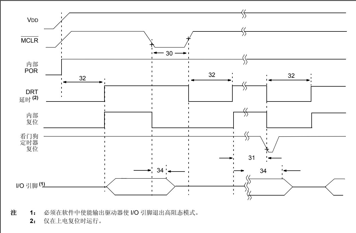
图 10-3: 复位、看门狗定时器和器件复位定时器时序
