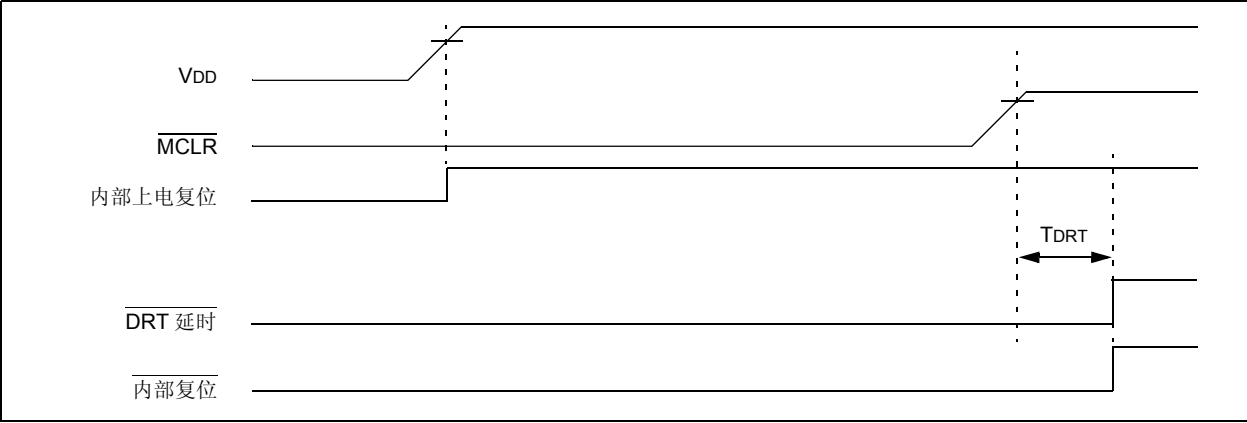
图 8-3: 上电延时时序 ( \overline{MCLR} 拉为低电平)
